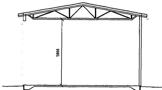
SEKTION - SKALA 1:100 -
