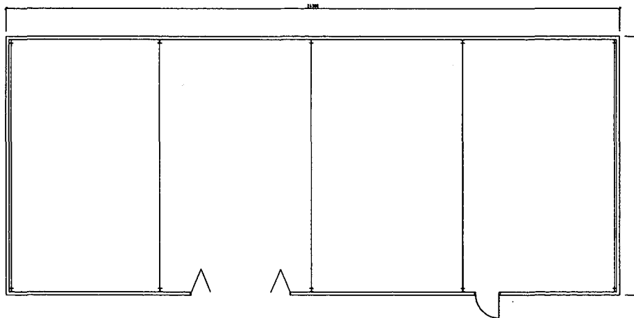
PLAN - SKALA 1:100 -
