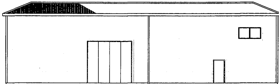
FASAD MOT NORR - SKALA 1:100 -
