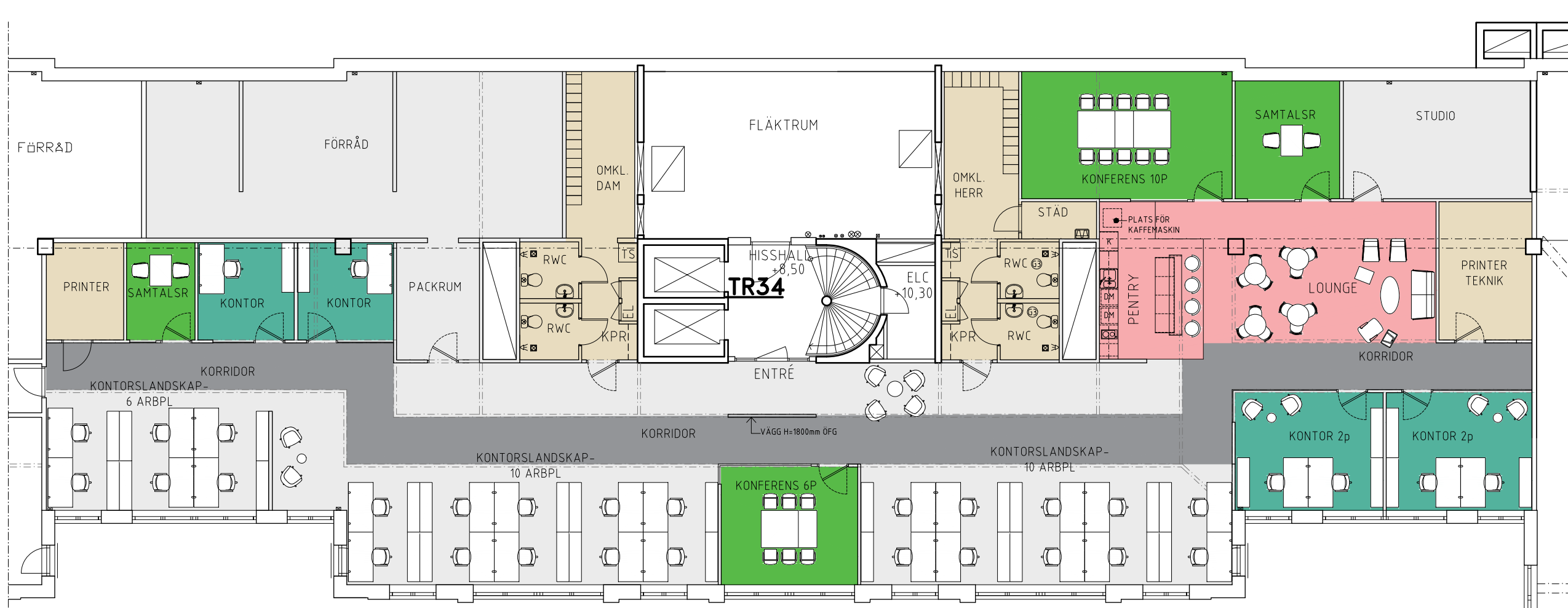
PLAN 1TR
