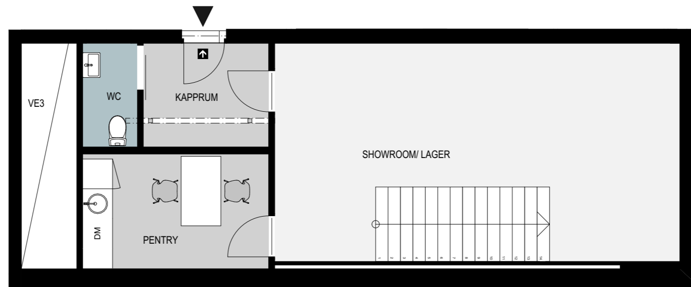
KÄLLARPLAN LOA 55kvm (TH 2,05m)
