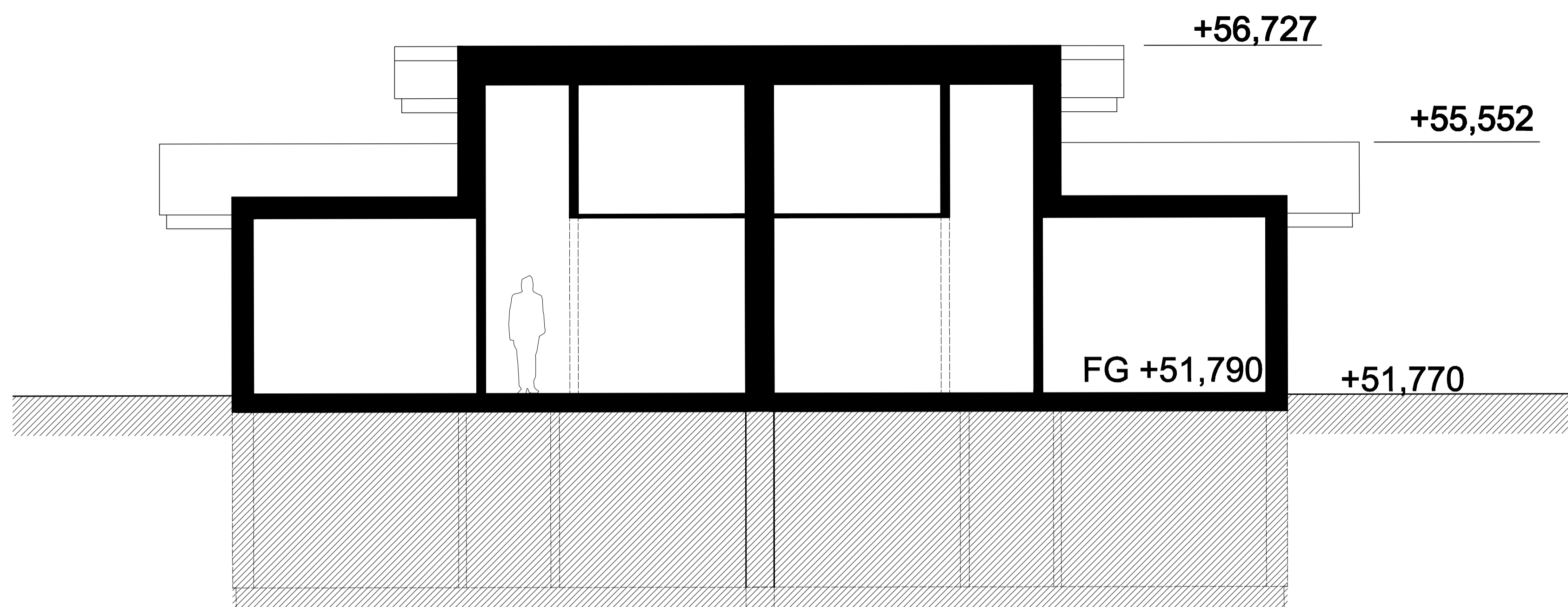
Sektion A-A
