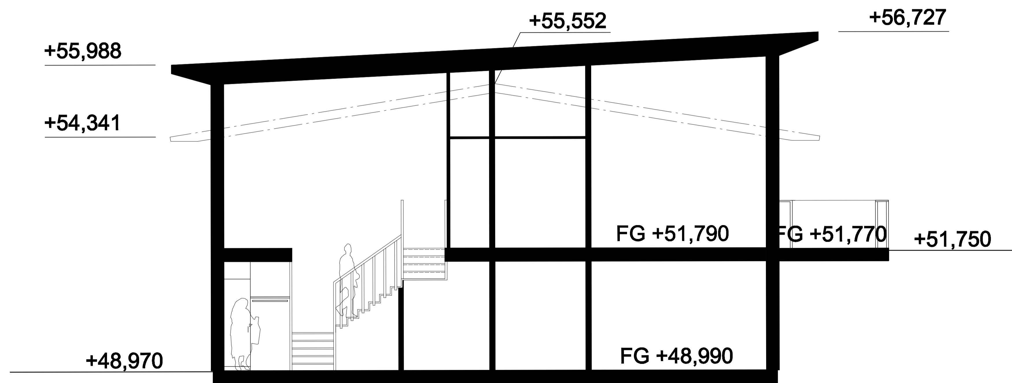
Sektion B-B
