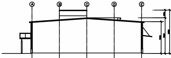
SEKTION B-B
