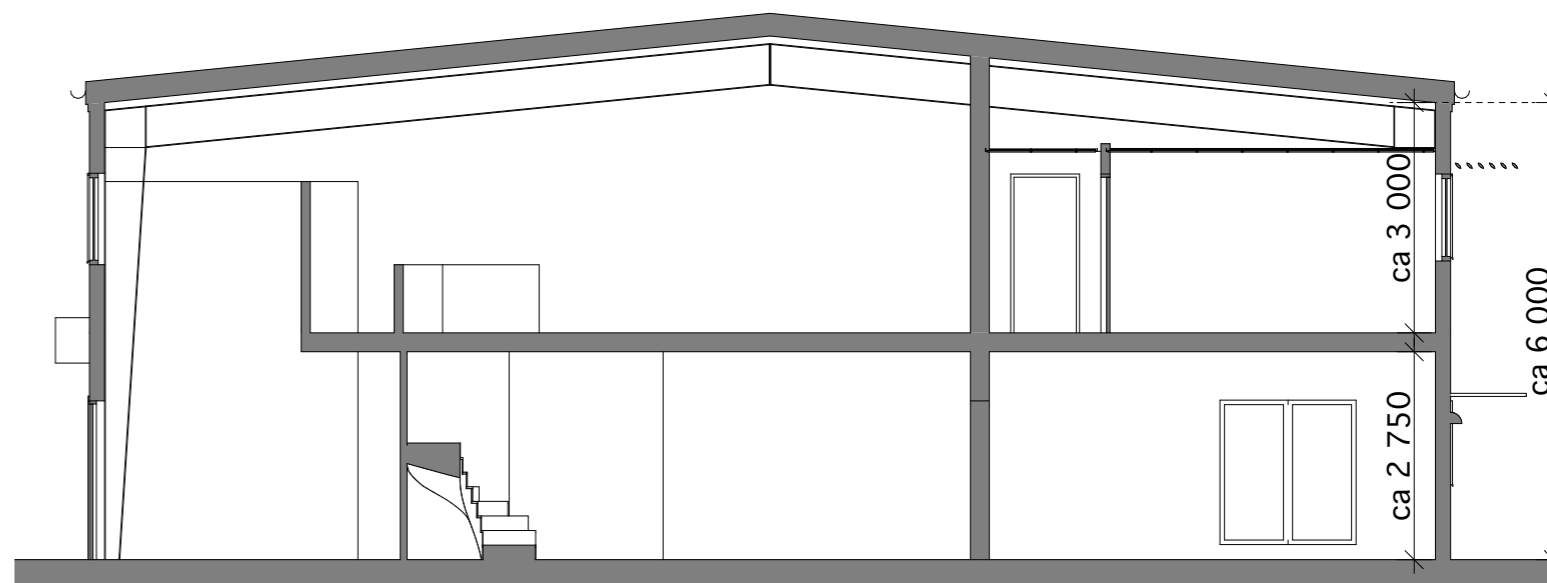
SEKTION A-A
