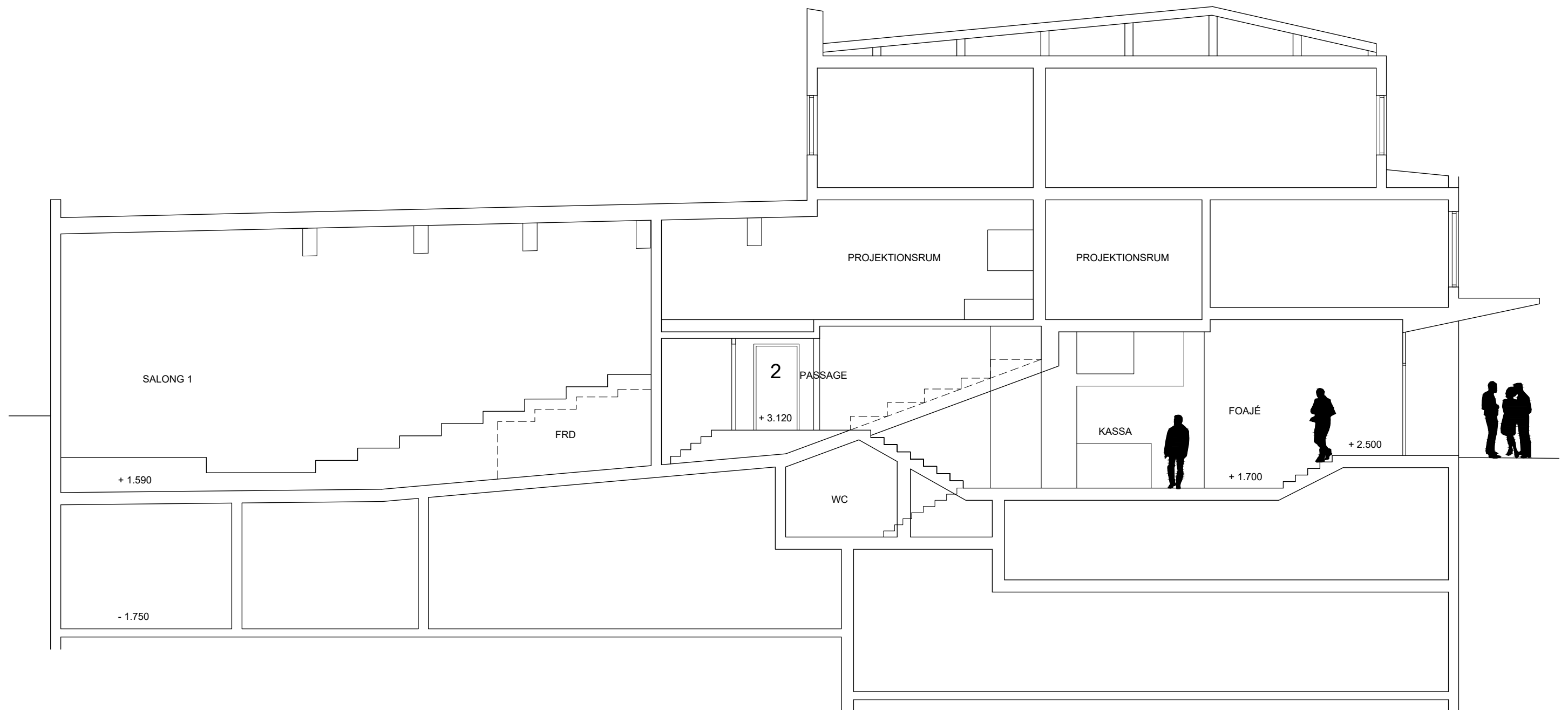
SEKTION A-A
