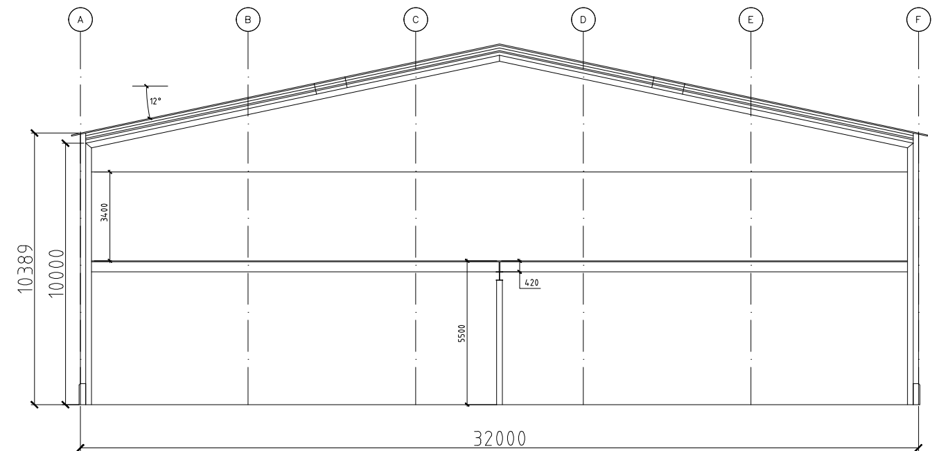
SEKTION A-A
