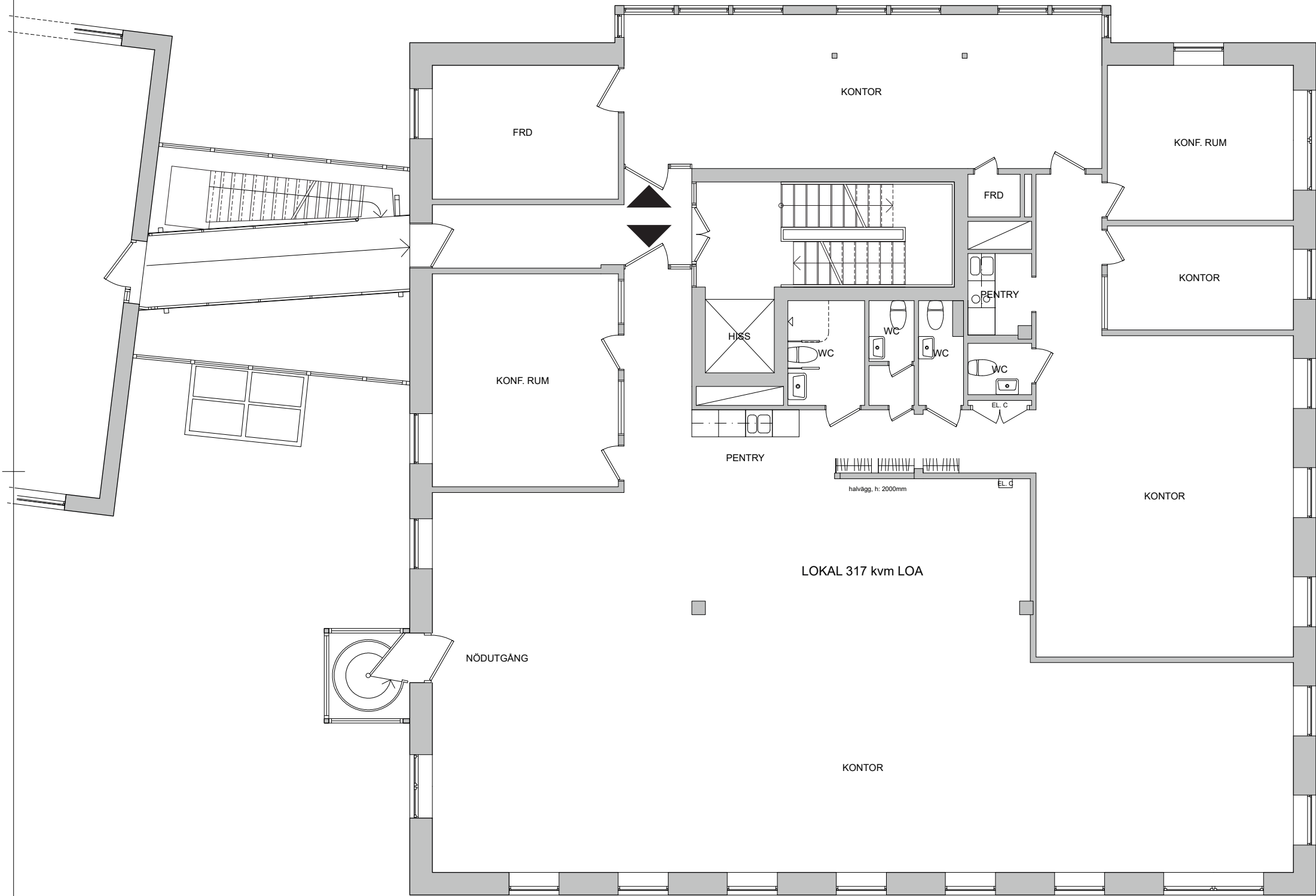
PLAN 01 1:100
