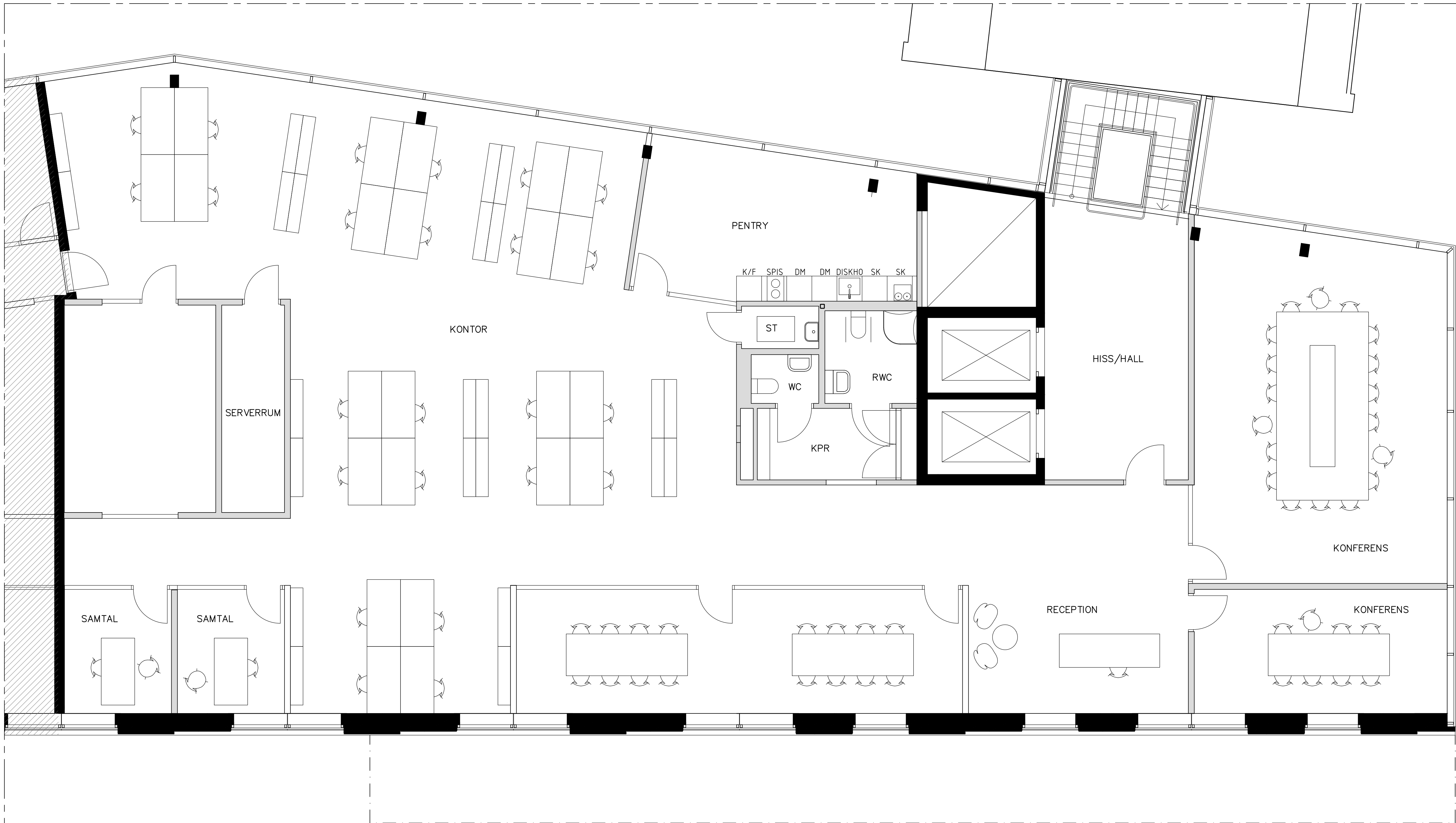
PLAN 6, DEL 2 1:50 / 1:100
