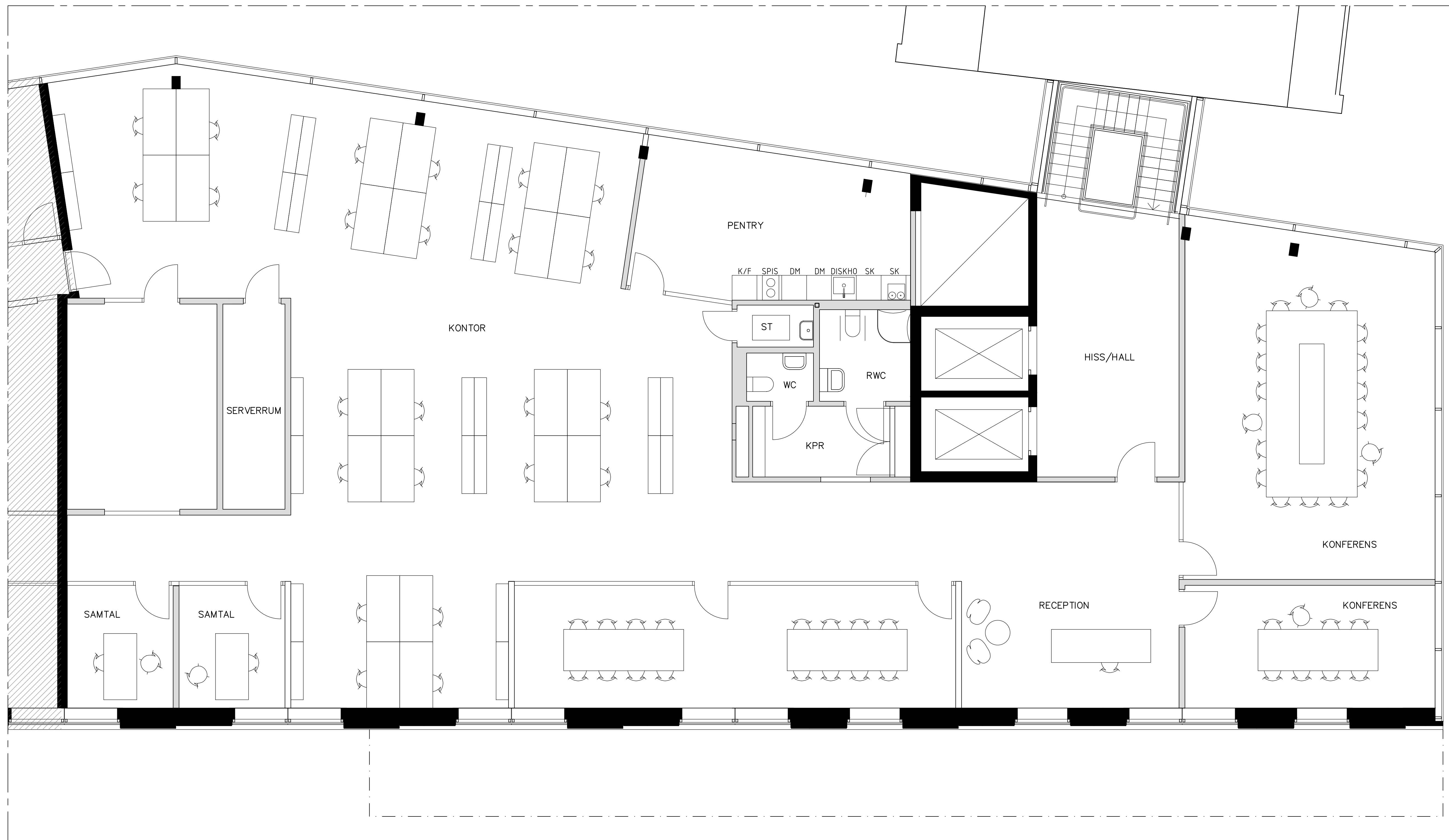
PLAN 6, DEL 2 1:50 / 1:100
