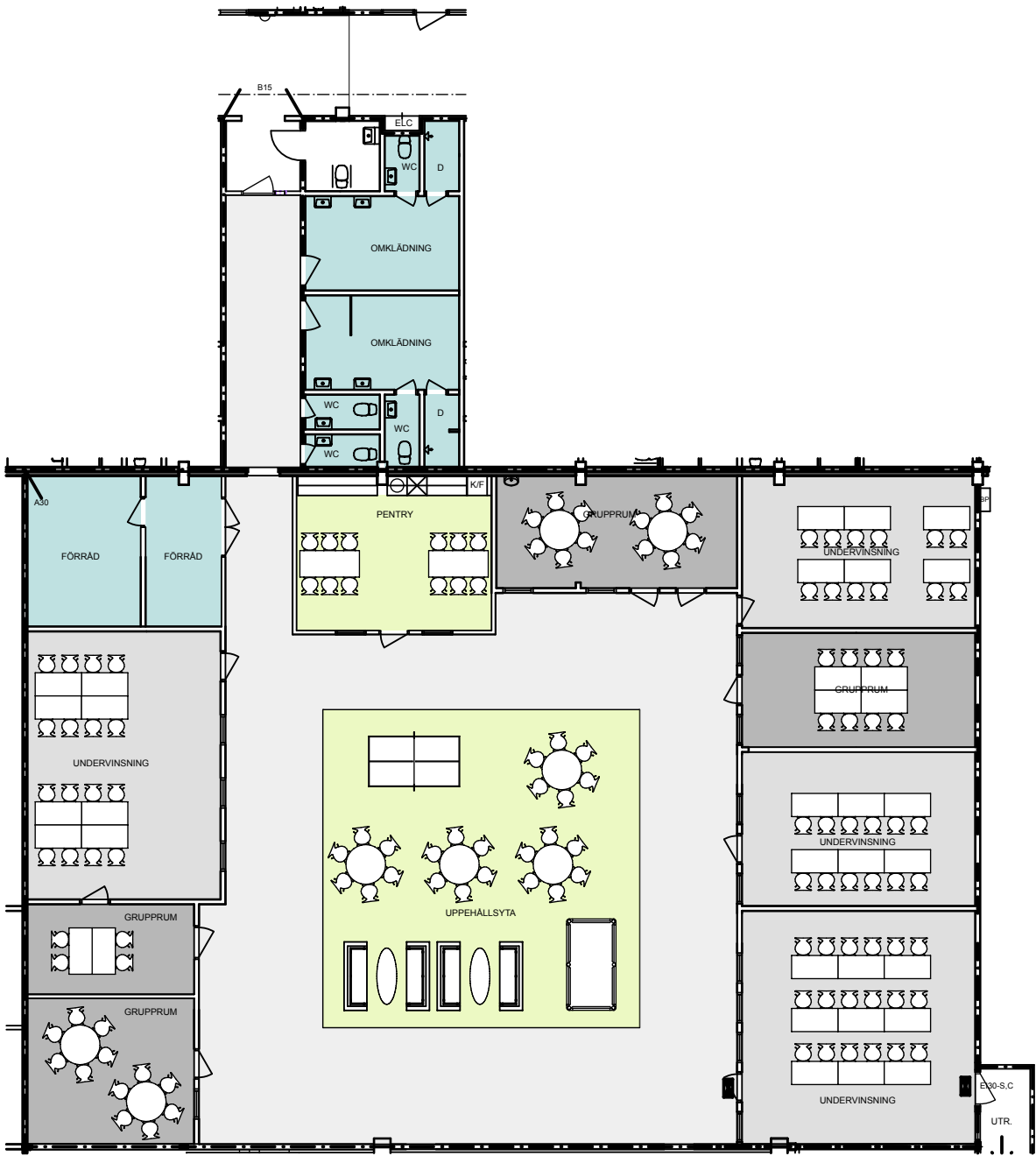
SKALA 1:200
