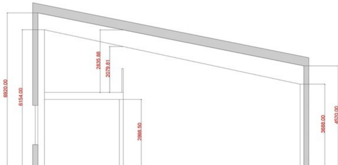
Genomskärningsbild över lager/produktions ytor med angivna höjdmått
