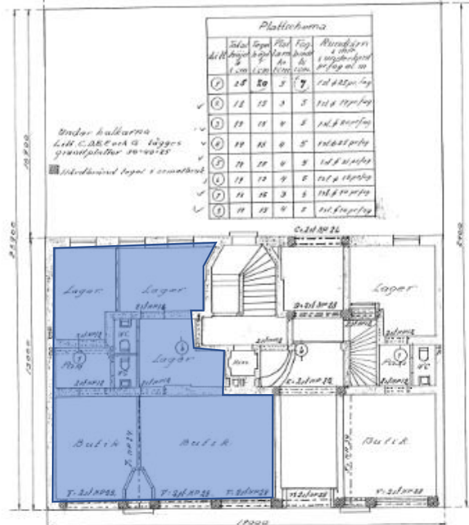
Plan av bottenvån.
