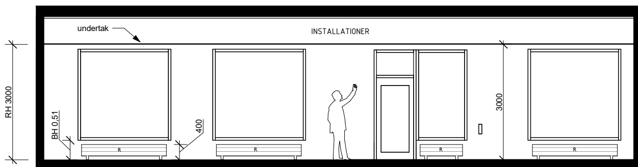
SEKTION B-B
