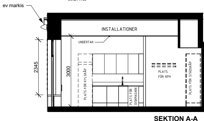
SEKTION A-A
