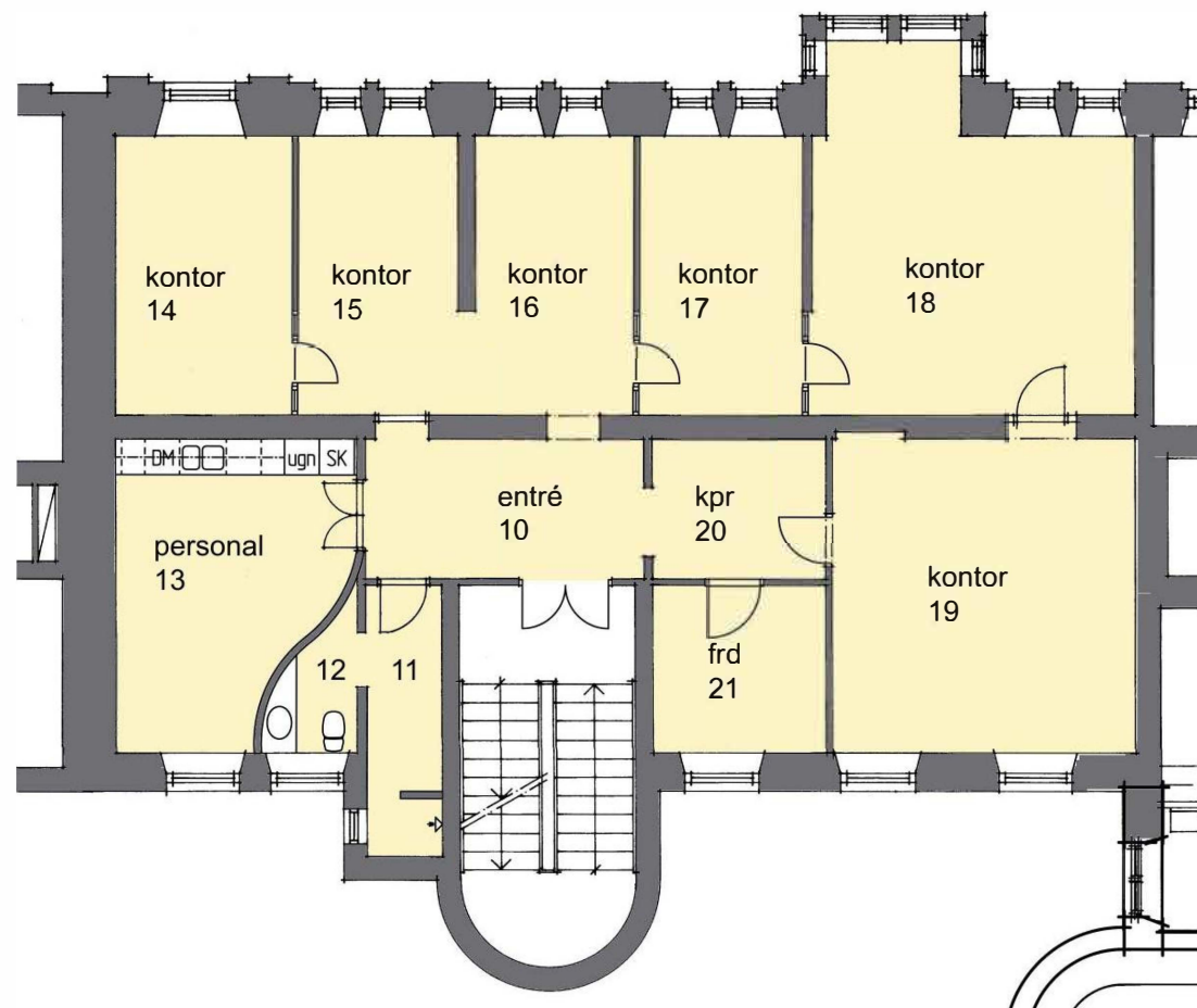
PLAN 1:100
