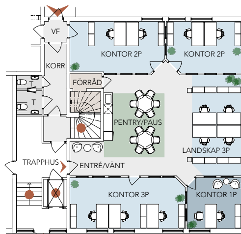
PLAN 1, BOTTENVÅNING
