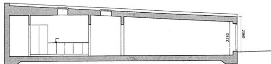
SEKTION A-A 1:100
