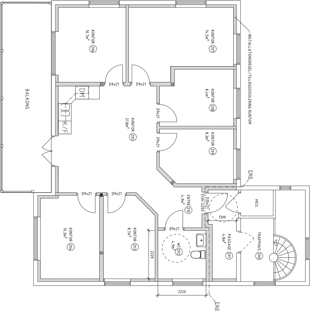
-PLAN 2 -1:100- (A3)
