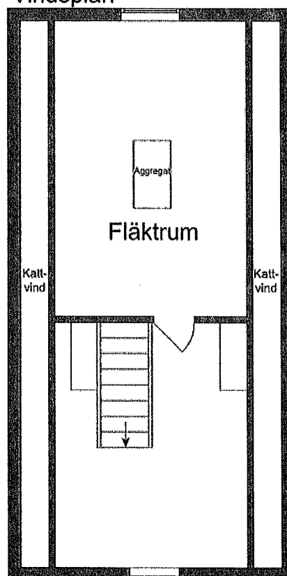
Vindsplan
