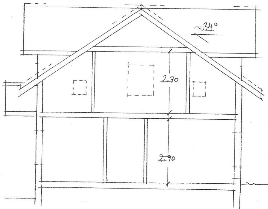
SEKSION A-A
