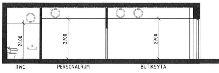
SEKTION A-A
