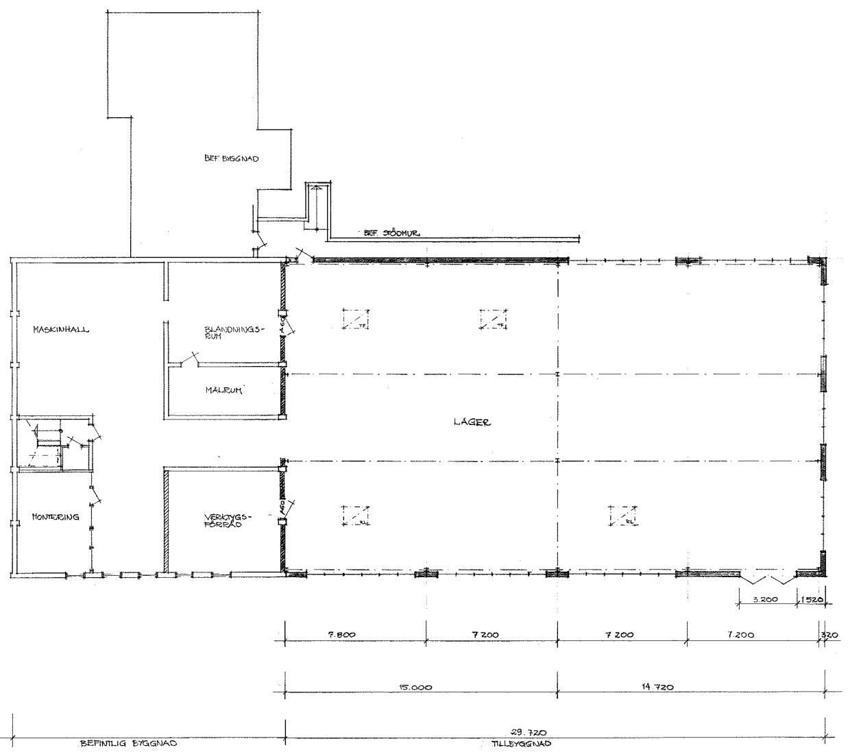
SUTERRÅNGPLAN SKALA 1:100
