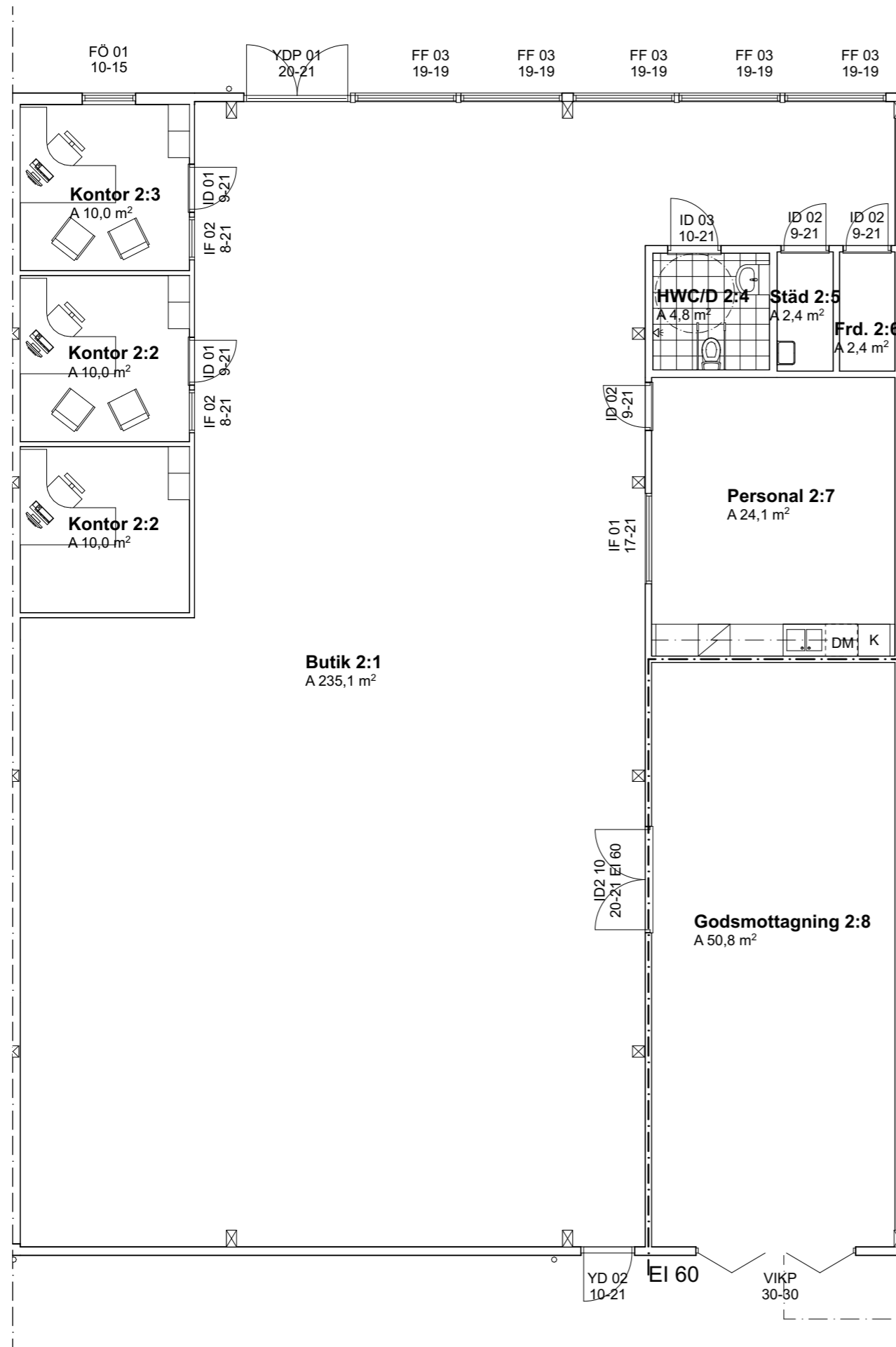
Plan 1 1:100
