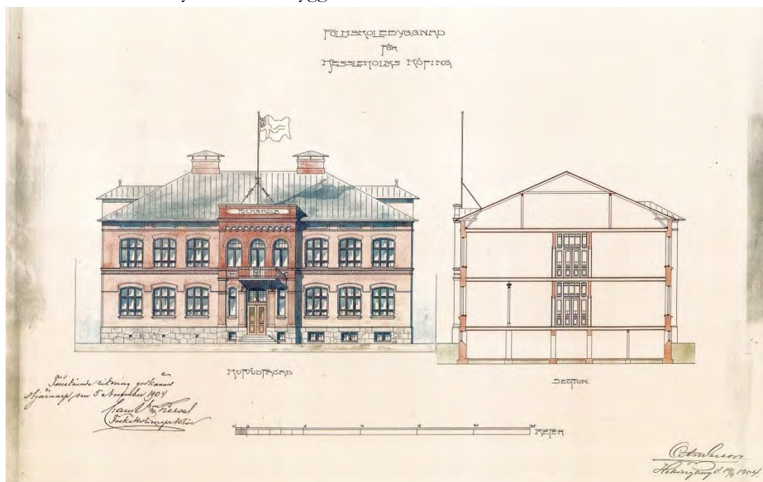
Figur 1 Originalritning kyrkskolan från 1905. Ritningen förvaras på kommunarkivet i Hässleholm.
