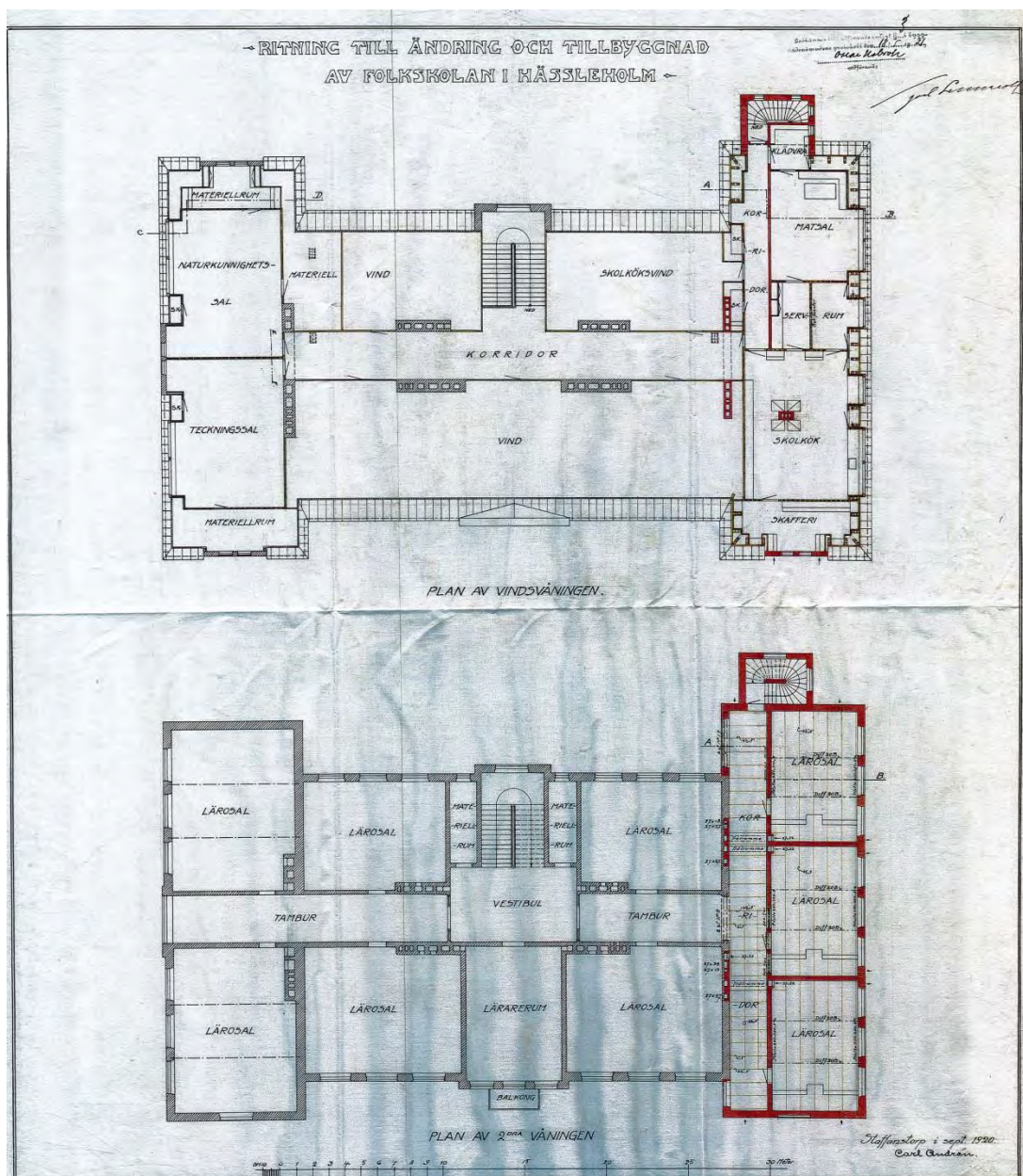
Figur 13 Ritning daterad 1920. Kyrkskolans andra våning och vindsvåning. Rödmarkeringen avser den planerade västra flygeln. På ritningen över vindsvåningen syns det materialrum där ett äldre väggfast skåp finns idag.
