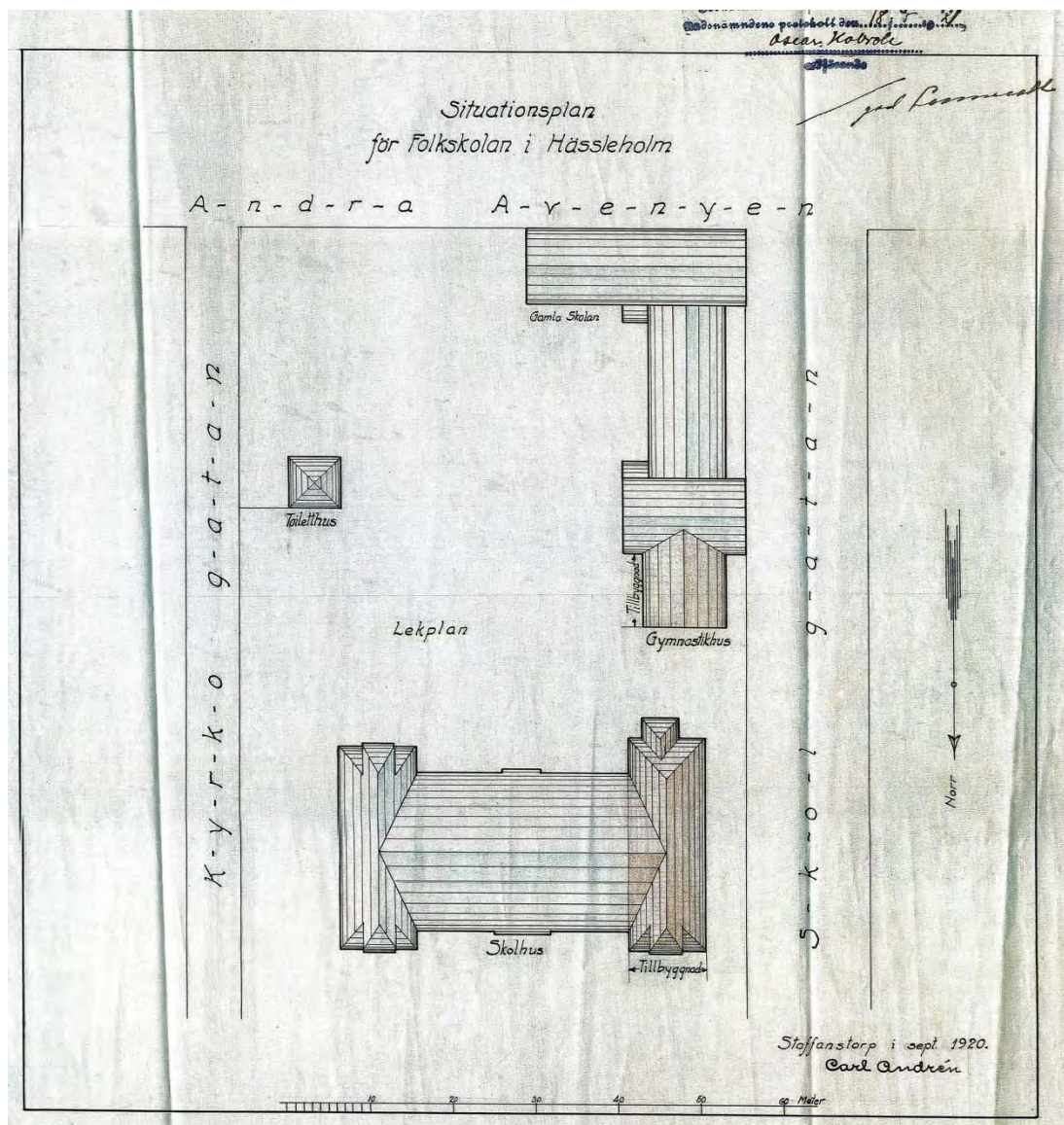
Figur 14 Situationsplan 1920. Här syns tillbyggnaden av omklädningsrum/duschrum på Folkskolan samt den tilltänkta västra flygeln på Kyrkskolan.
