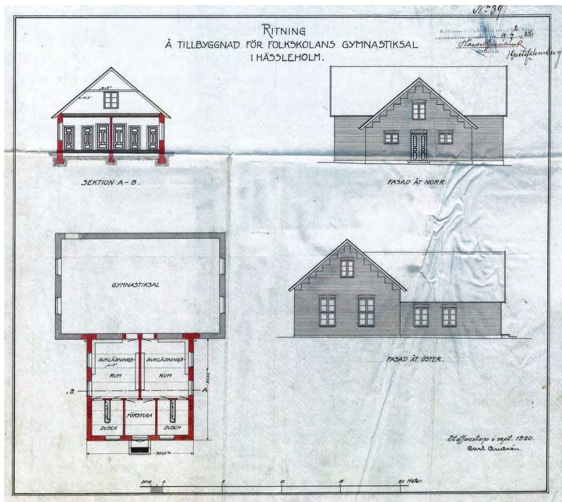
Figur 15 Tillbyggnad av omklädningsrum och duschrum vid folkskolans gymnastiksal.
