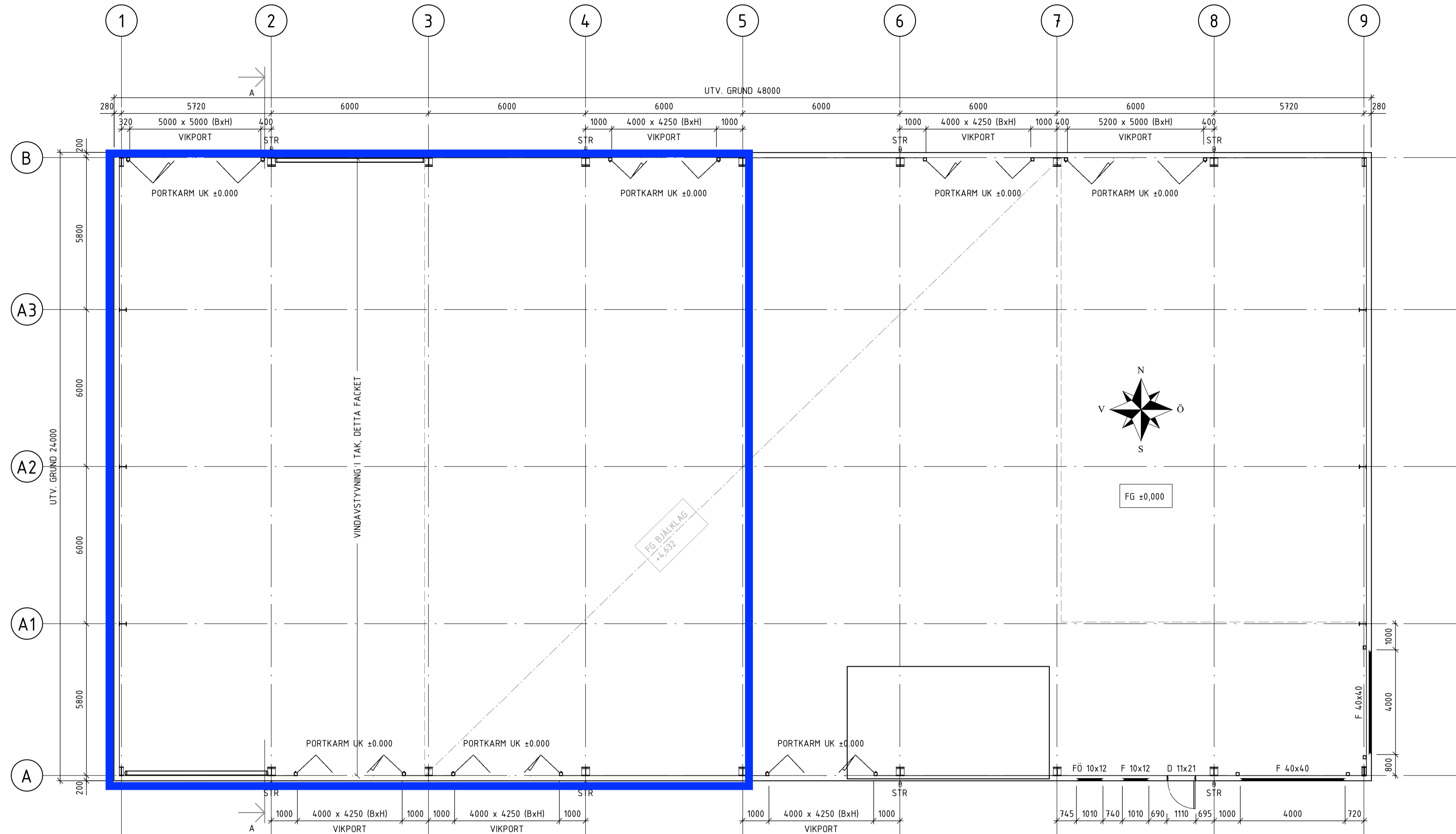
PLAN 1 1 : 100
