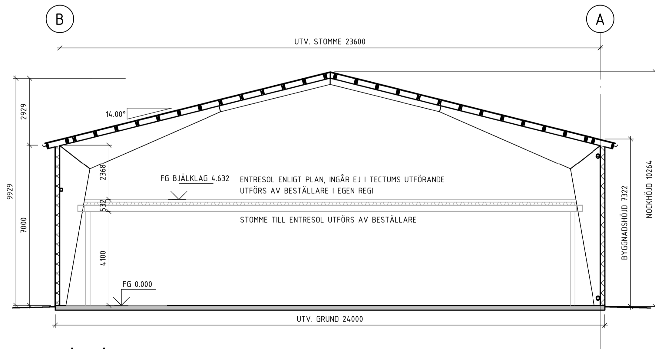
A - A 1 : 100
