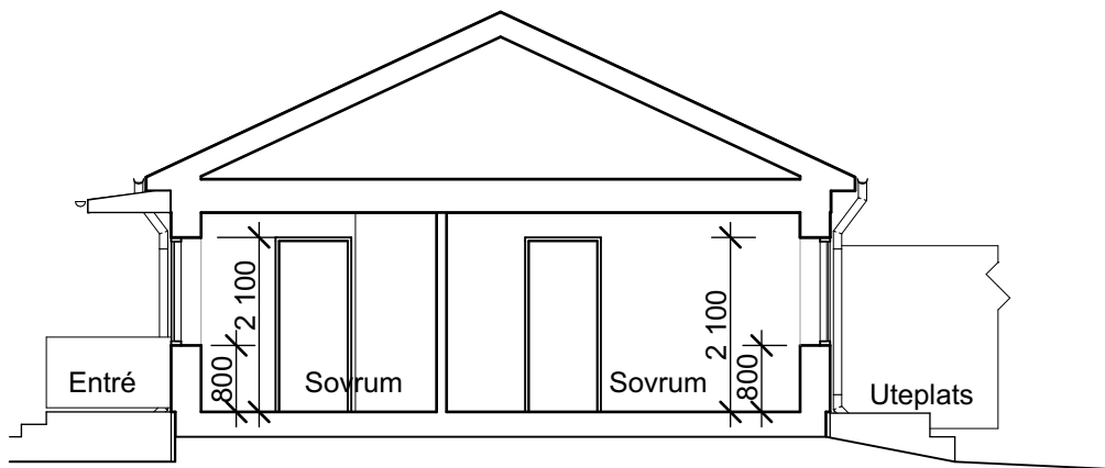
SEKTION B-B
