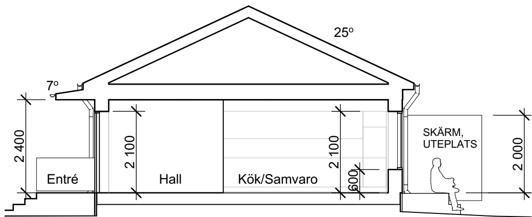
SEKTION A-A
