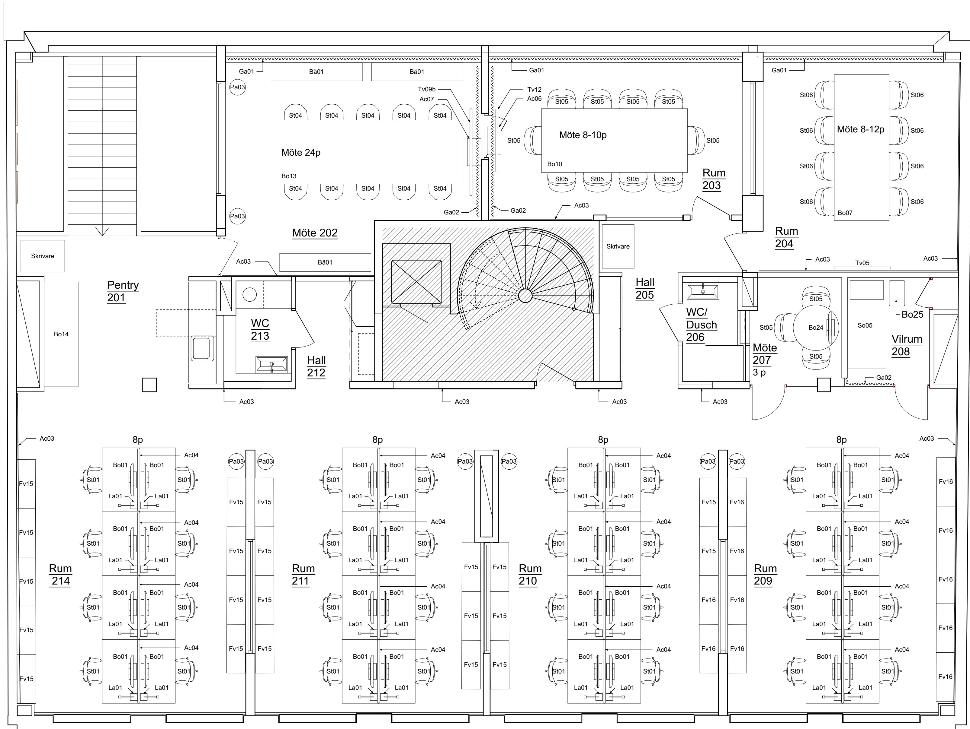
PLAN 2 1:50
