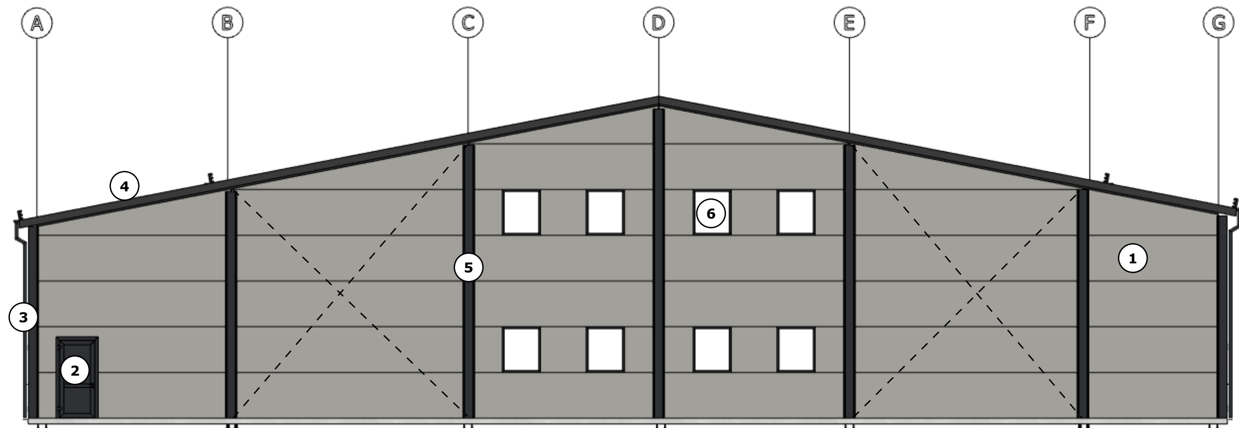
FASAD MOT NORDOST
