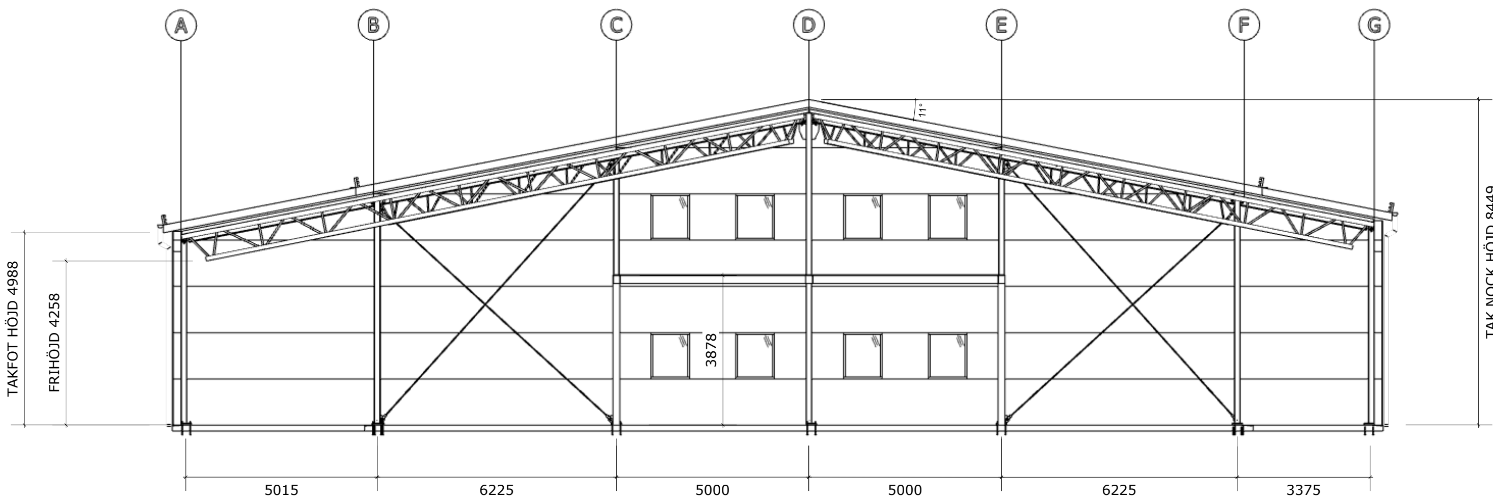
A-A
