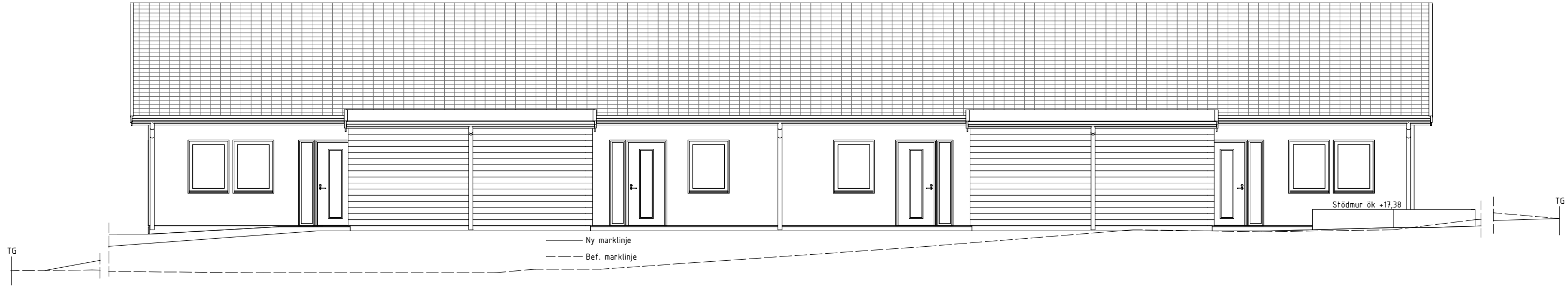
1 Fasad mot Norr Förråd 1 : 100
