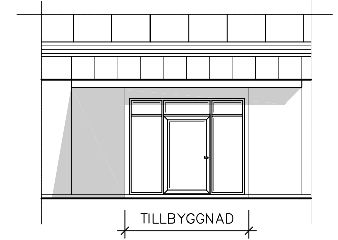
FASAD MOT SÖDER SKALA 1:100
