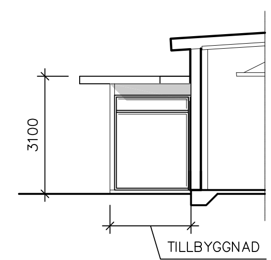
FASAD MOT ÖSTER SKALA 1:100
