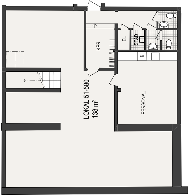
KÄLLARPLAN
