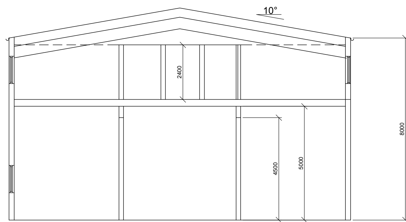
SEKTION C-C
