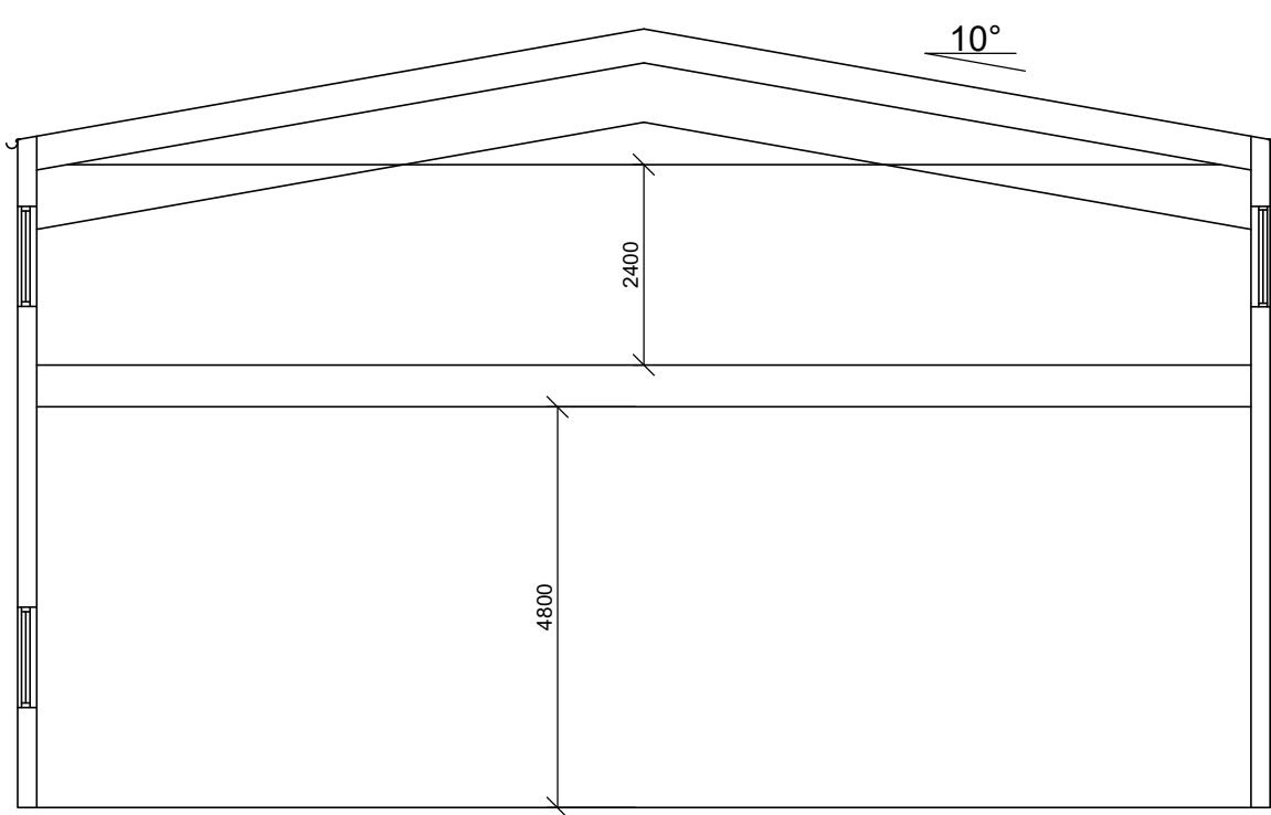
SEKTION B-B
