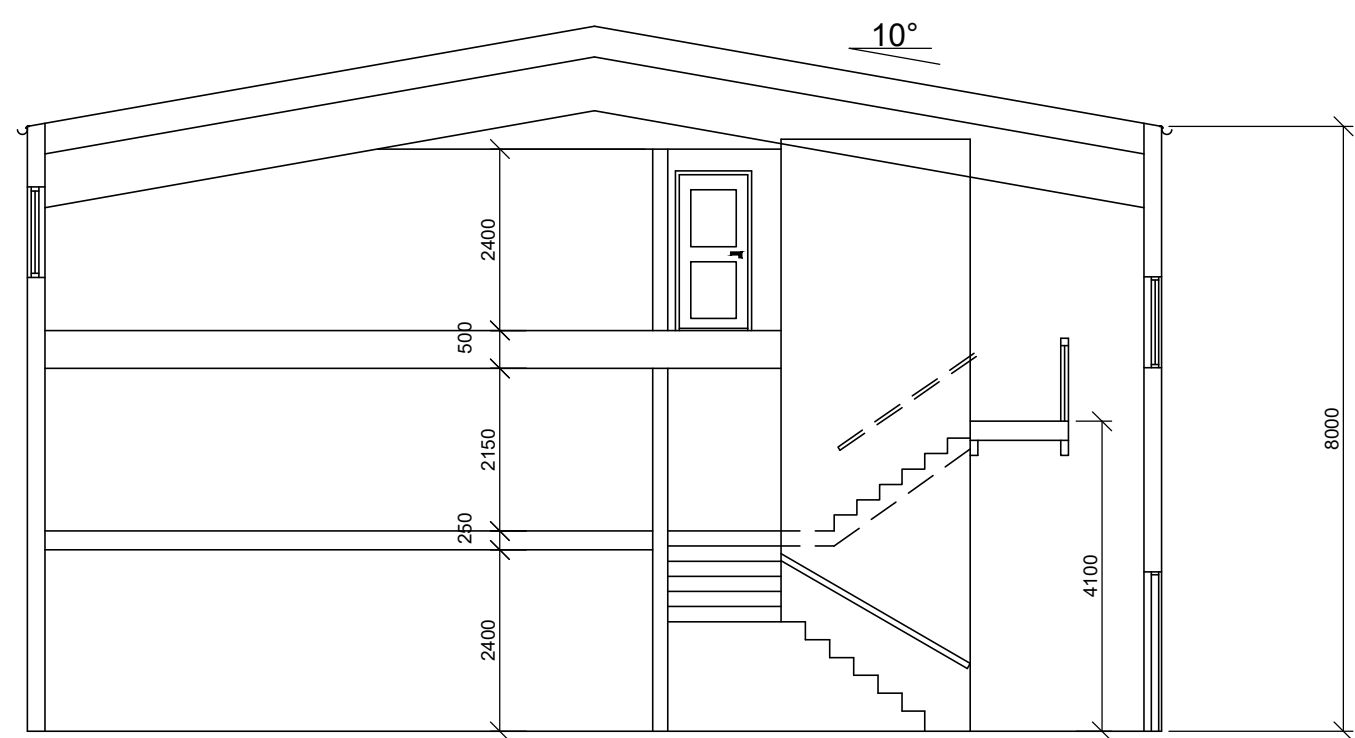
SEKTION A-A
