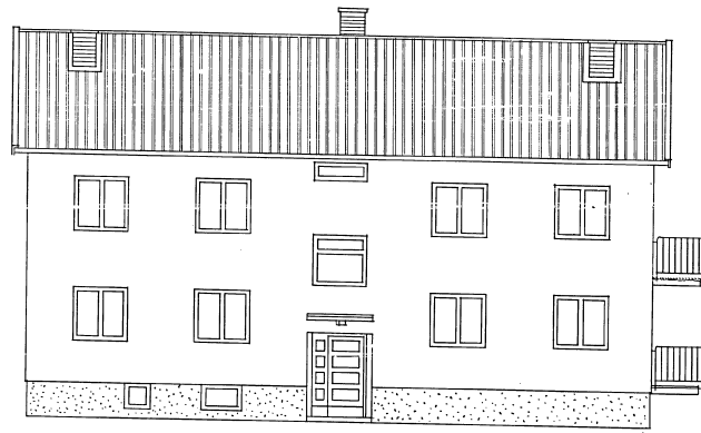
FASAD MOT NORDVÄST
