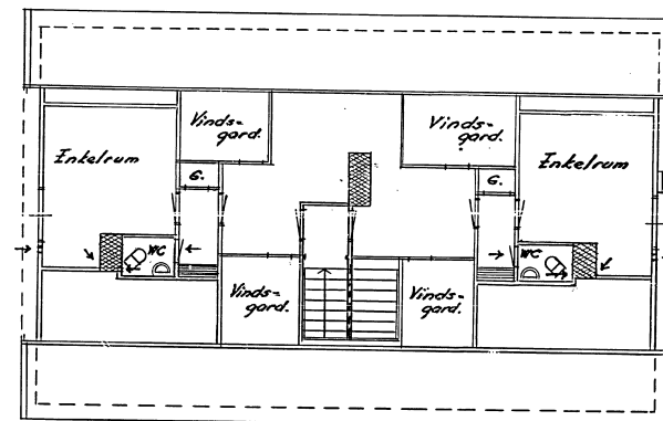
PLAN AV VINDEN
