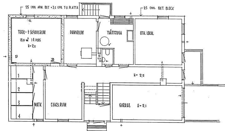
PLAN AV KÄLLAREN
