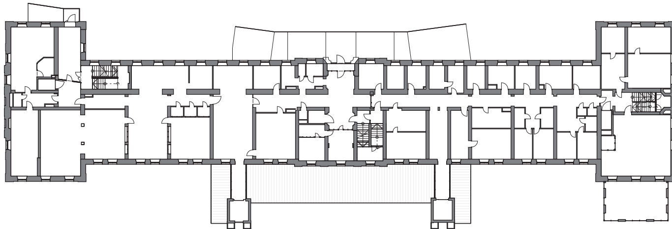
PLAN 5 (ÖVRE ENTREVÅNING)
