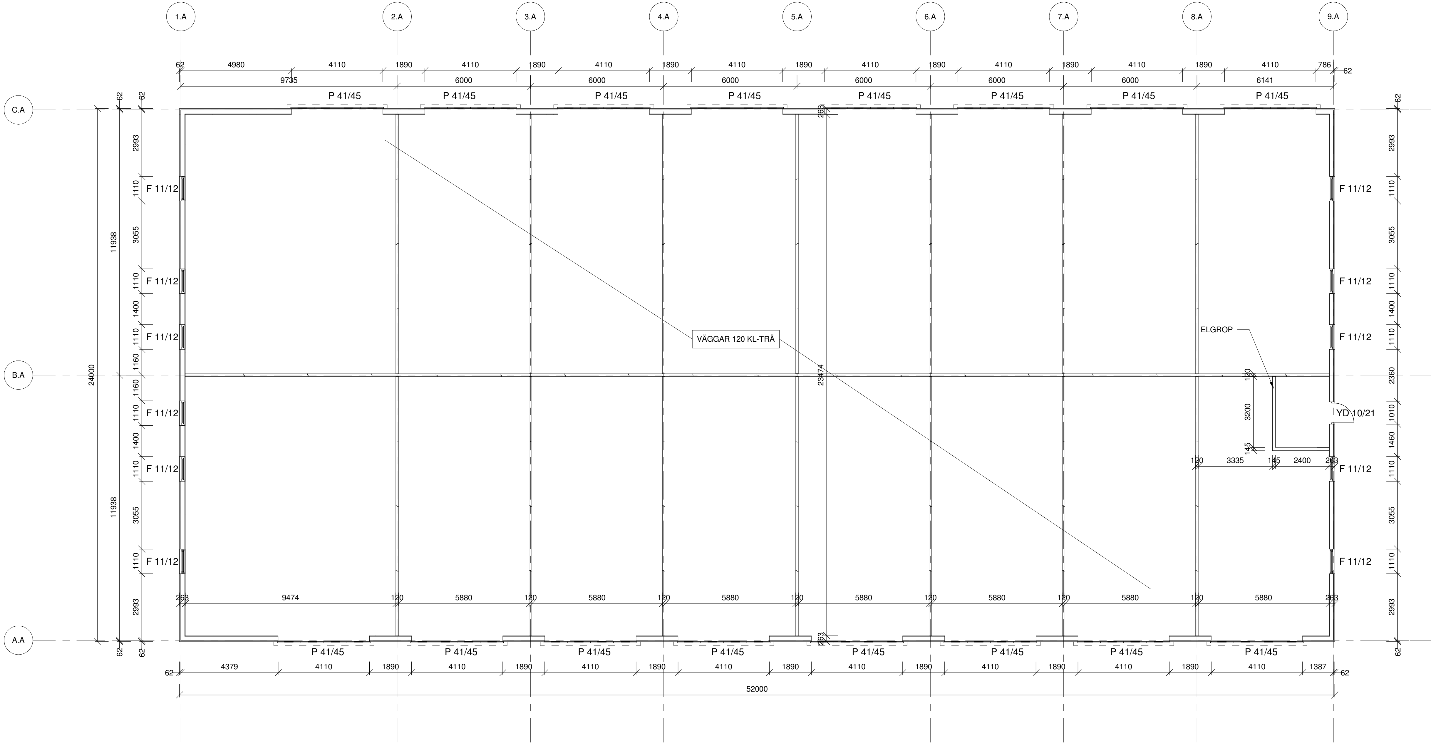
Plan Hus A 1 : 100
