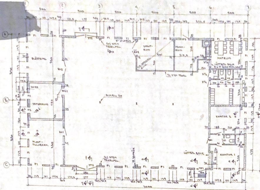
PLAN, 1:100
