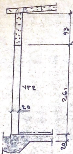
SEKTION 1-1 1:50
