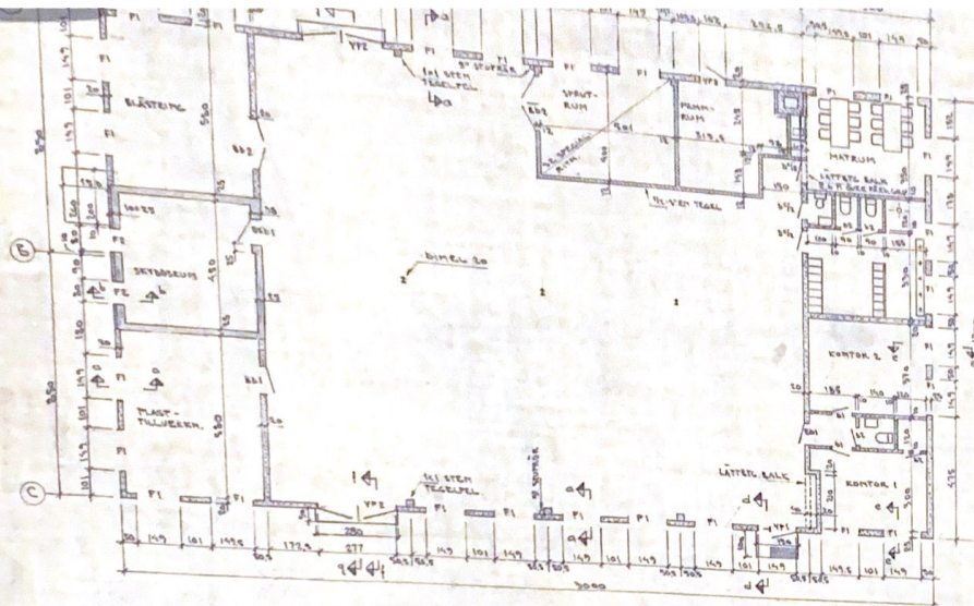
PLAN, 1:100
