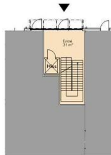
Plan 1, Entréplan 1:200
