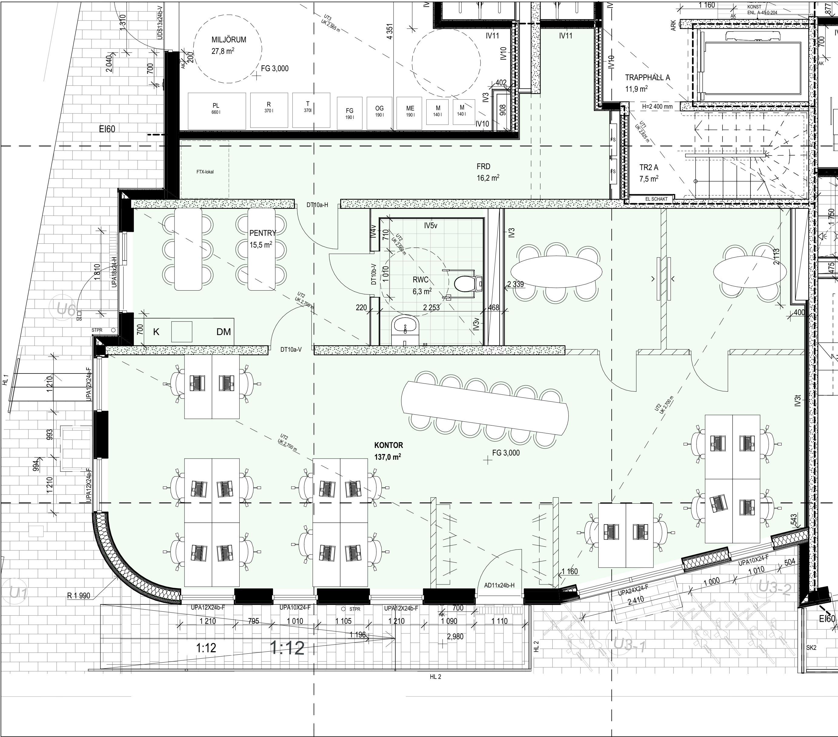
Kontor 1:50
