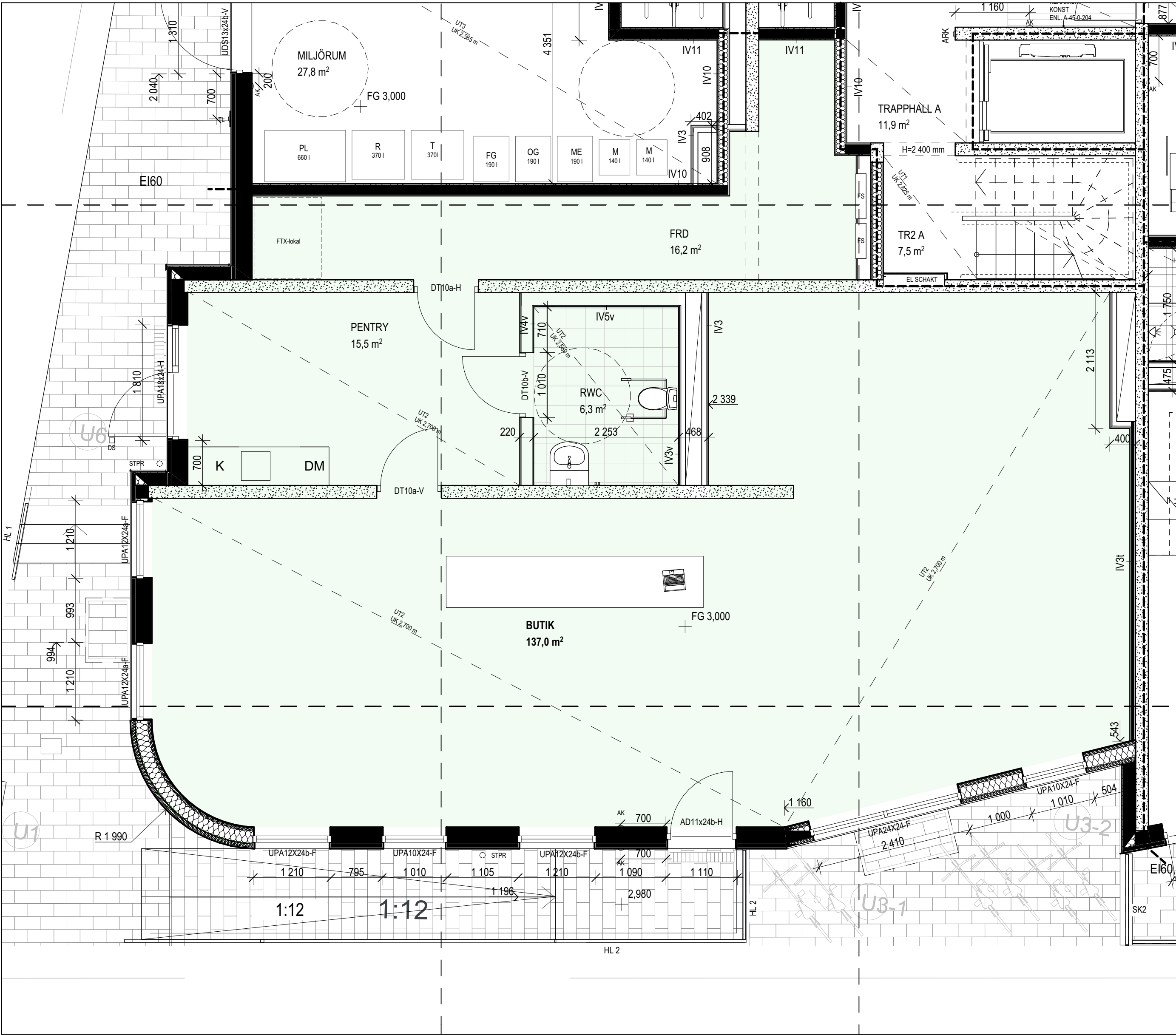
Butik 1:50
