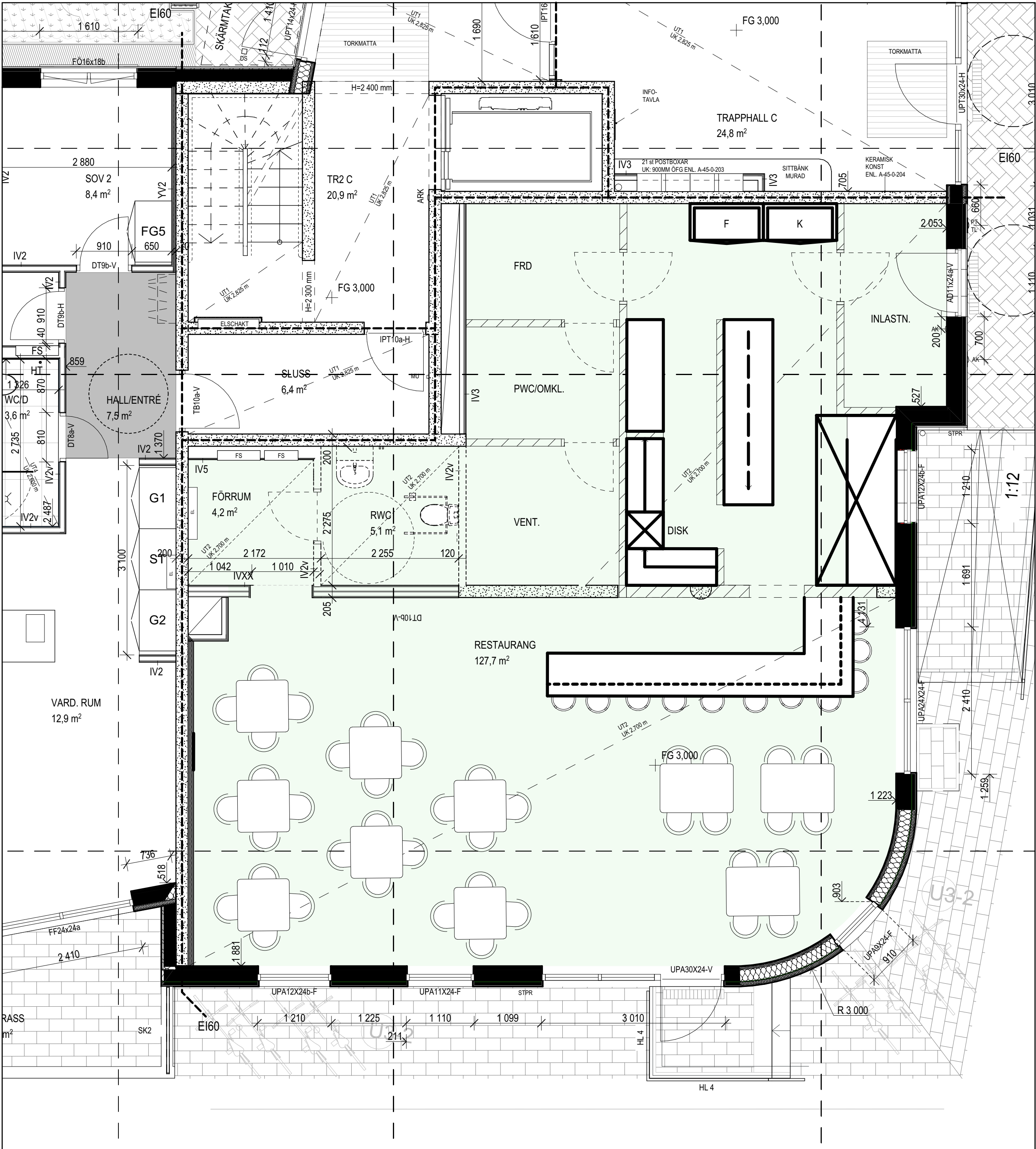
Exempel 2, Restaurang layout 1:50
