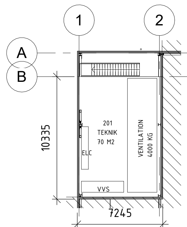
2 Entresolplan - Lokal A 1 : 200
