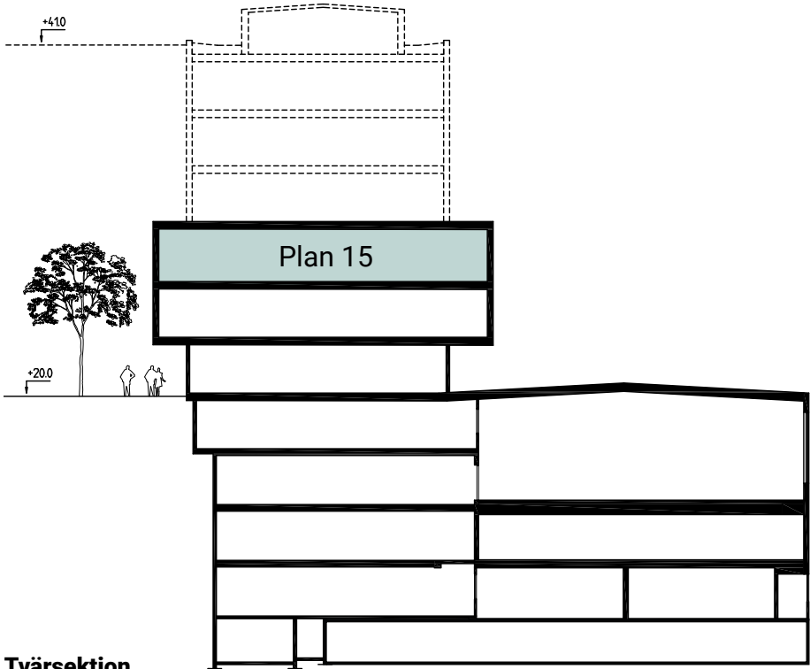
Tvärsektion Skala 1:400
