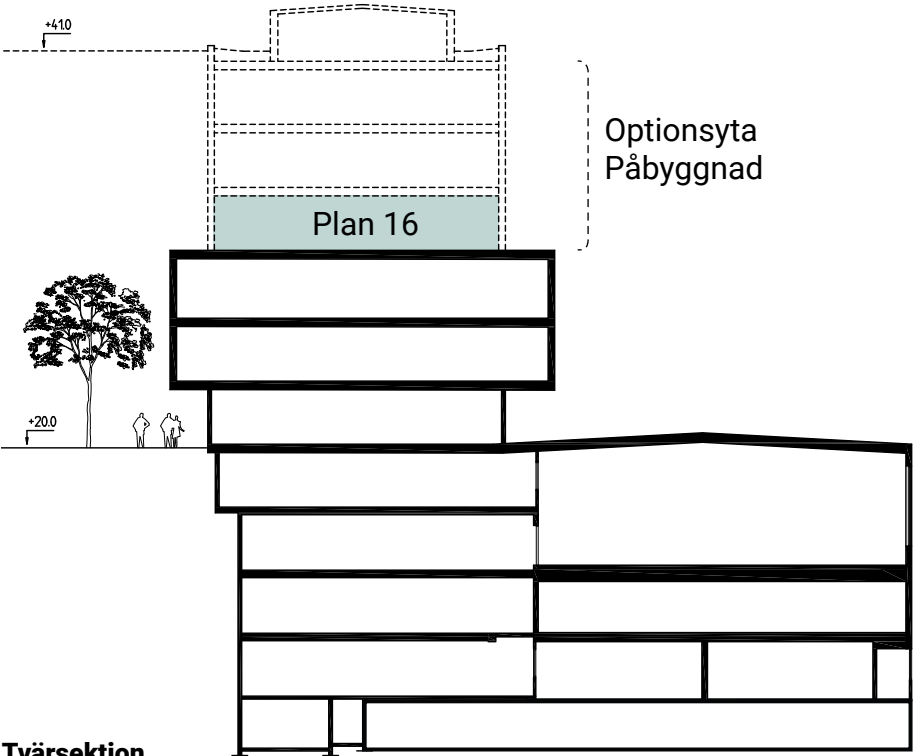
Tvärsektion Skala 1:400
