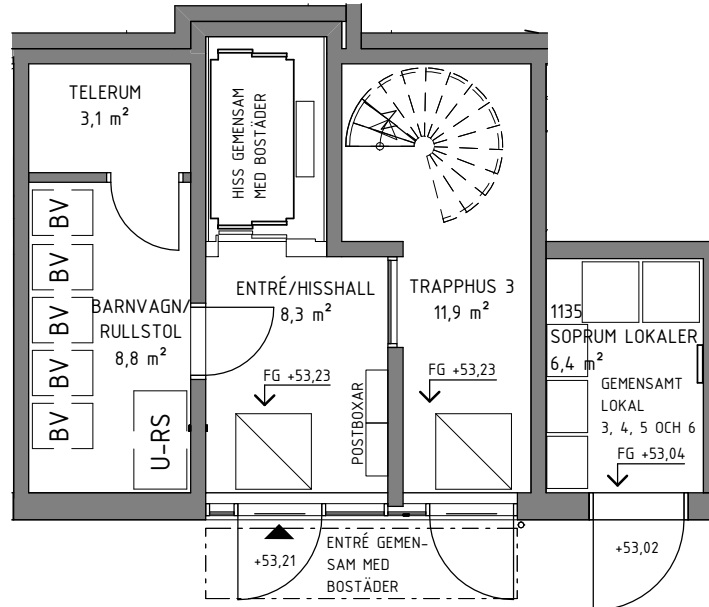
PLANVY ENTRÉPLAN
