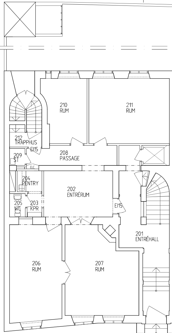
ÖVRE ENTRÉVÅNING
