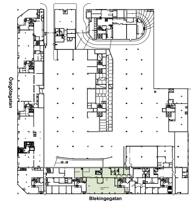
Översiktsritning
