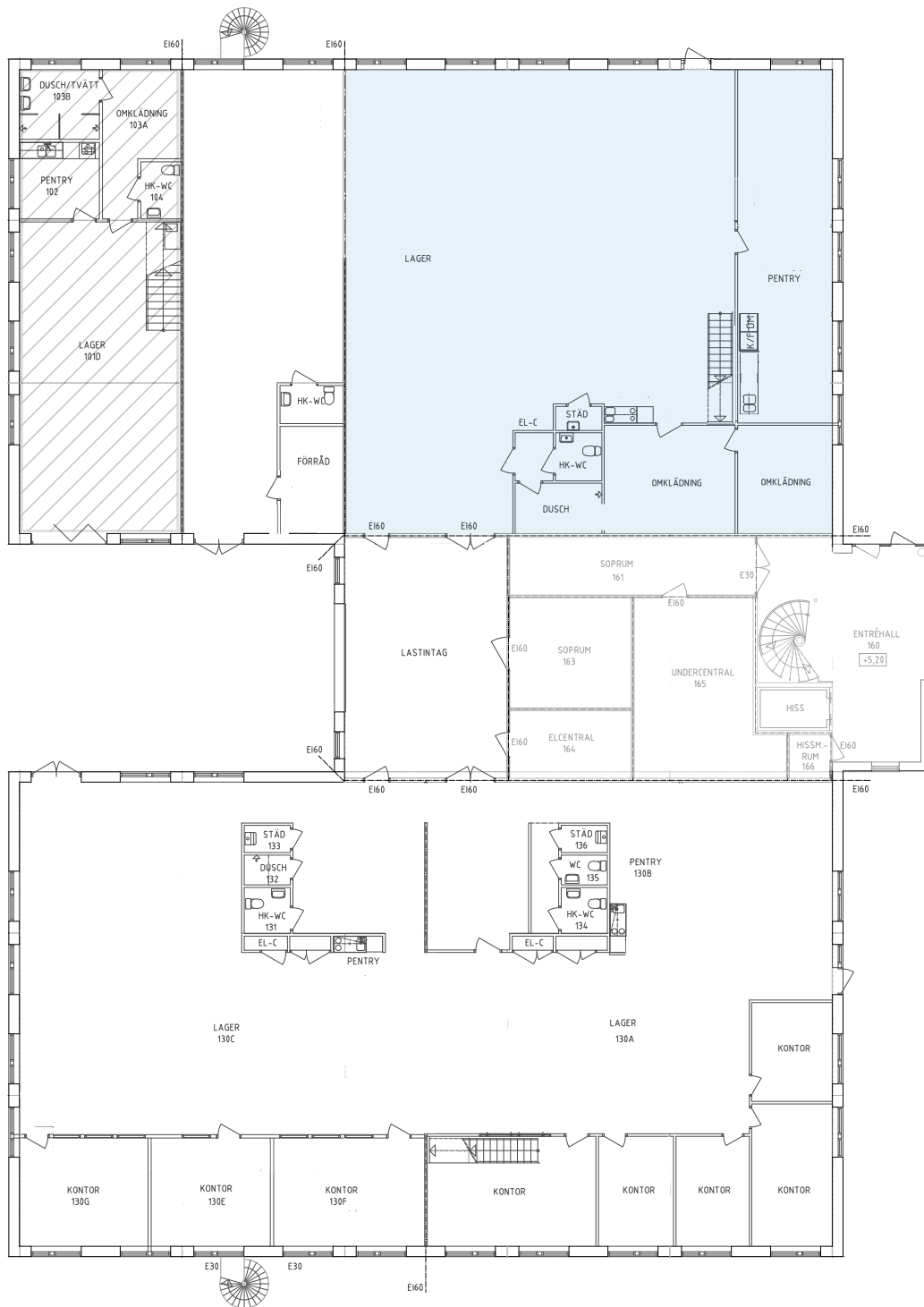
Plan E Kv ROTFJÄRILEN 1 PLAN 0, ENTRÉPLAN
