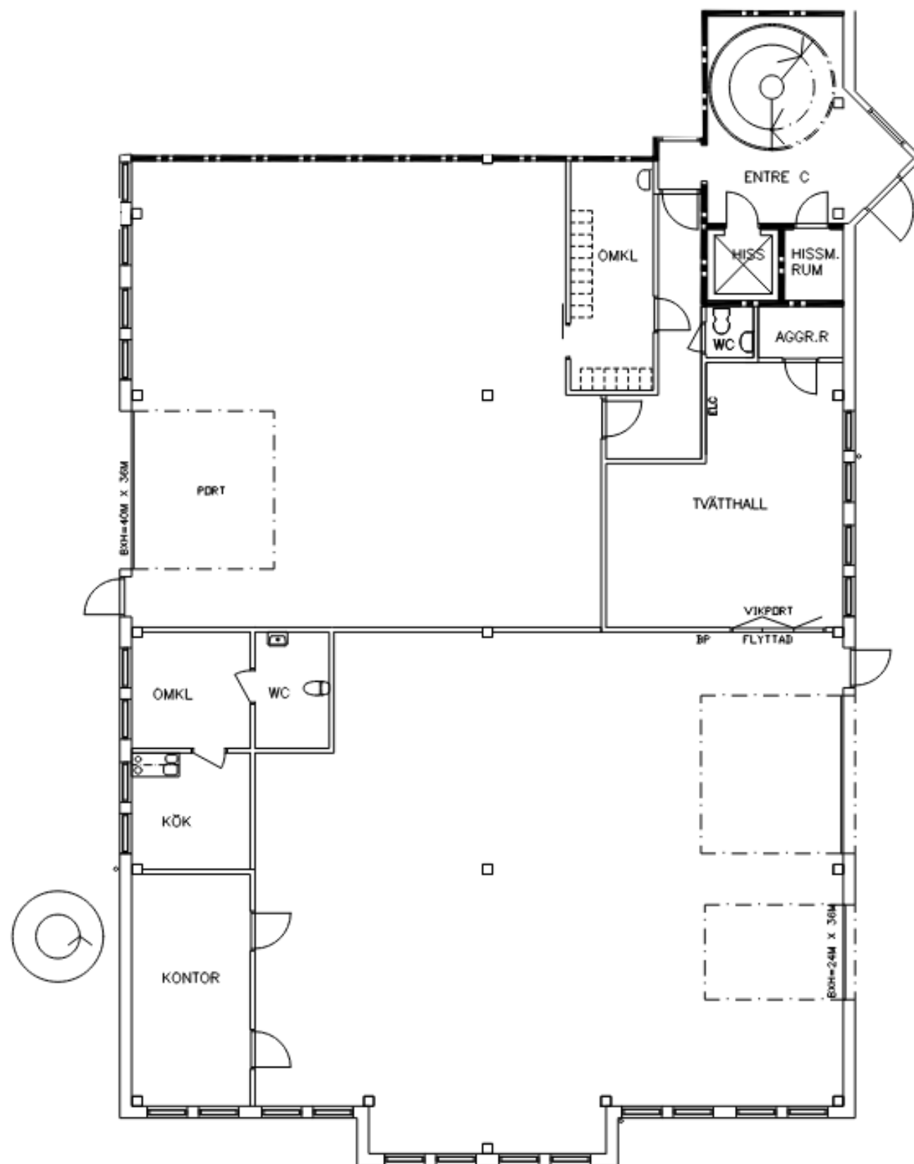
PLAN 0 LAGER/VERKSTAD - 426 KVM
