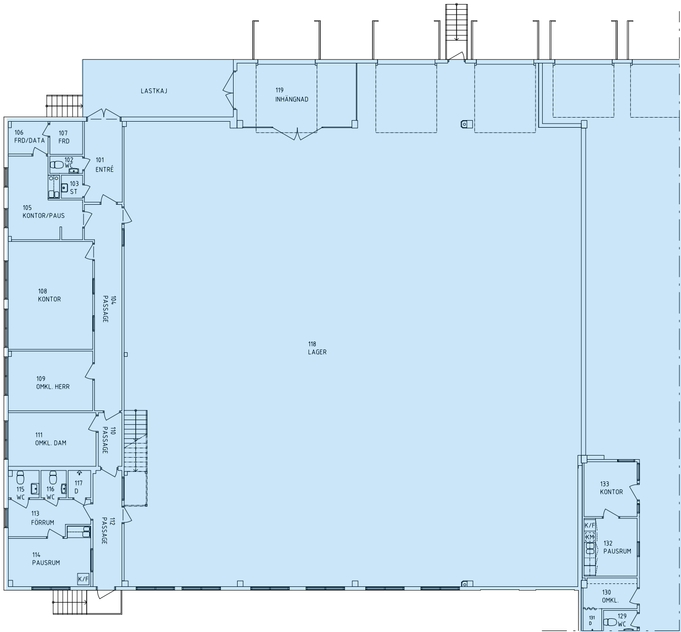
BOTTENVÅNING, DELPLAN 1:200
