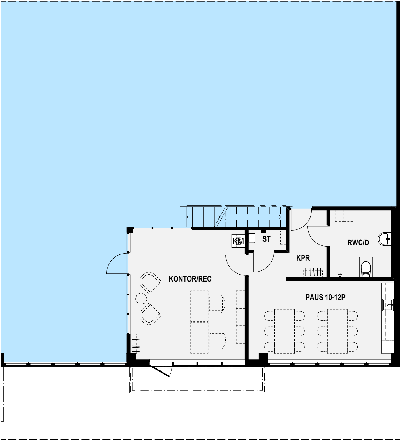
PLAN 1, KONTOR & PERSONALYTOR
