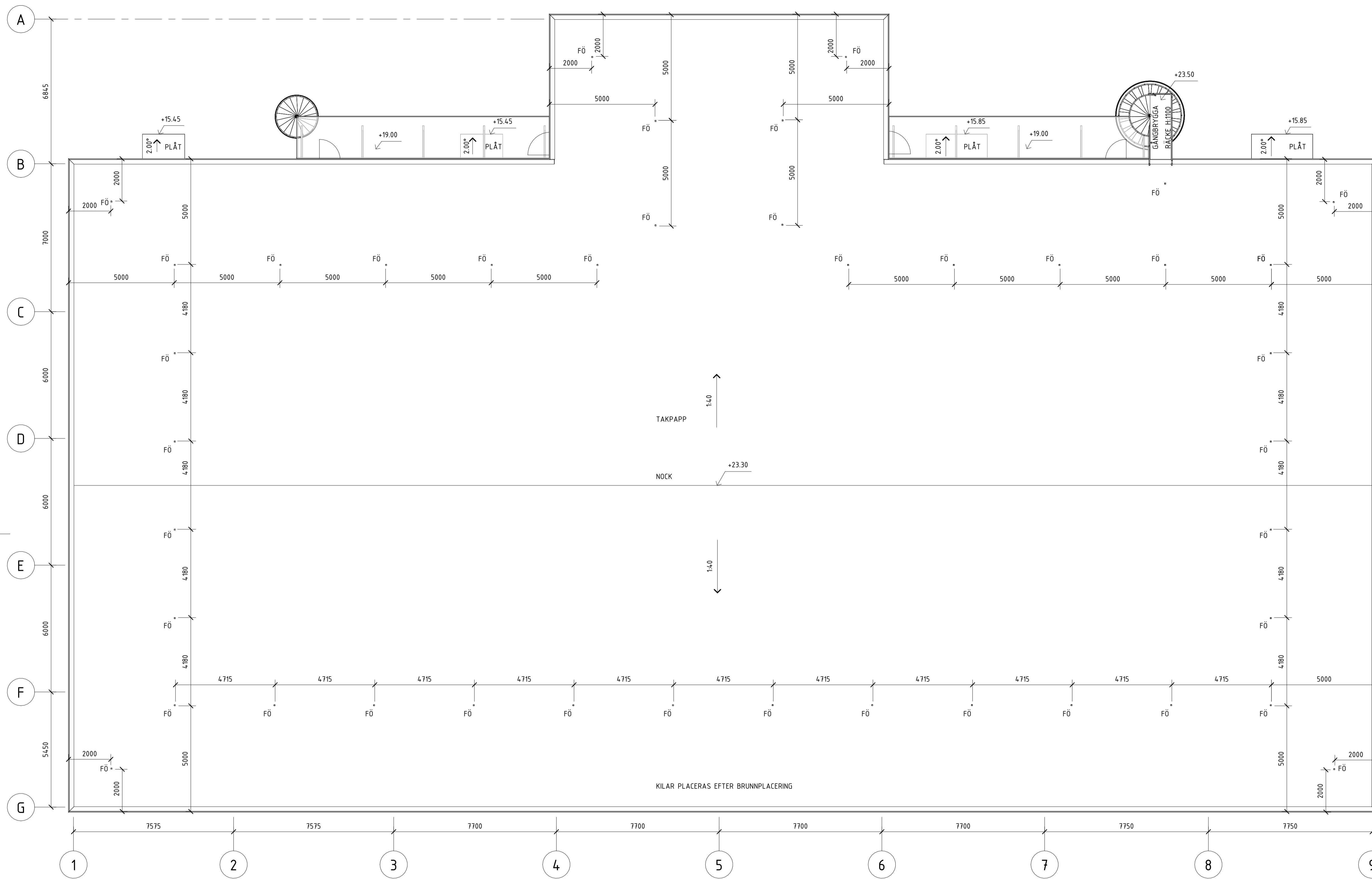
TAKPLAN SKALA 1 : 100
